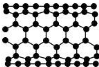
Рисунок 2 — Изображение фрагмента ОУНТ со структурой типа «кресло»
