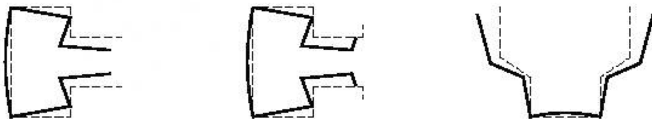
Рисунок 15 — Потеря устойчивости сечения сложной формы
