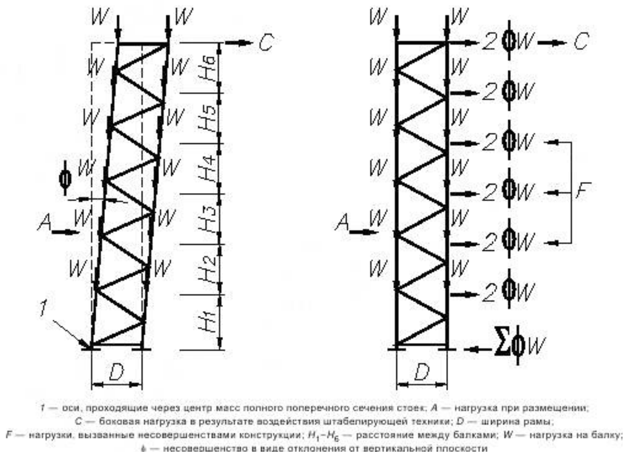
Рисунок 30 — Расчетная схема для расчета на устойчивость в Y-направлении конструкций стеллажа с крестовыми раскосами жесткости
