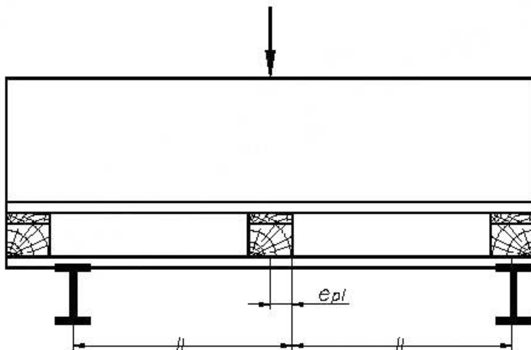
Рисунок Е.1 — Эксцентриситет нагрузки
