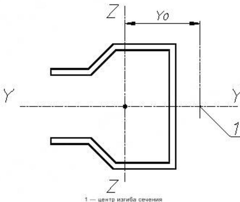
Рисунок 23 — Центр изгиба сечения
