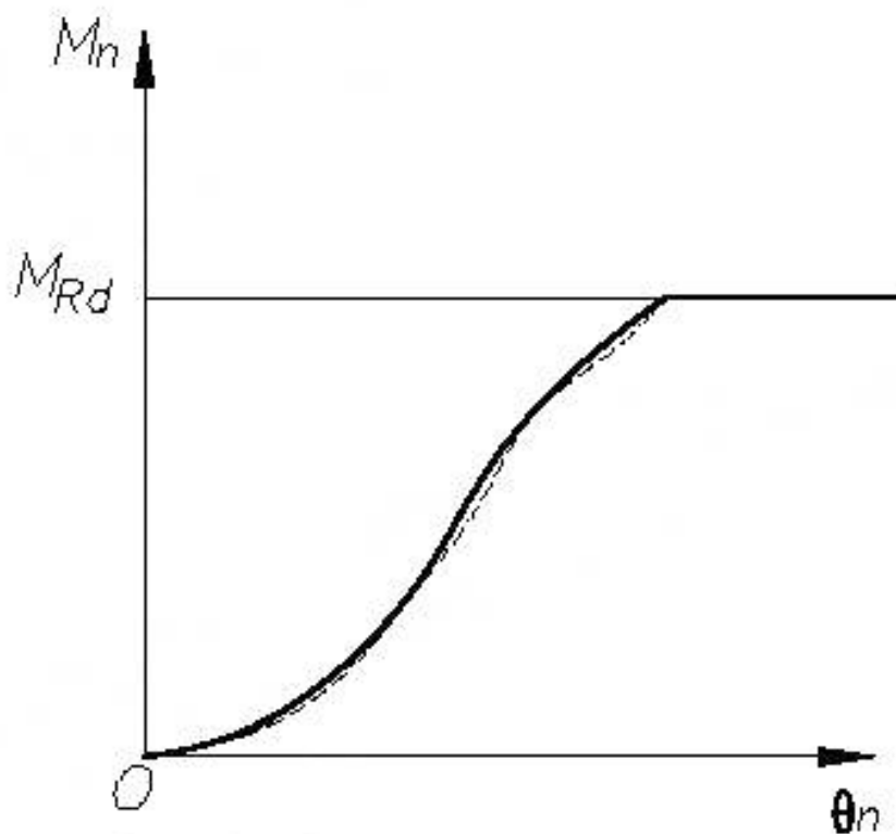
Рисунок А.8 — Типовая линеаризация средней кривой
