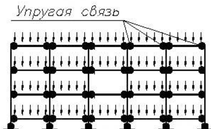
Рисунок 27 — Схемы нагружения для расчета в X-направлении
