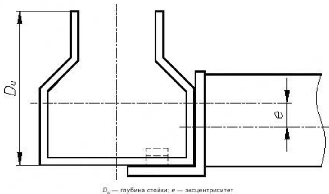
Рисунок 11 — Эксцентриситет в Y-направлении
