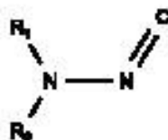
Рисунок В.8 — Молекулярная структура нитрозамина
