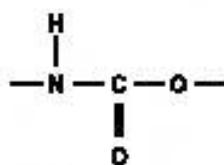
Рисунок A.1 — Уретановые группы
