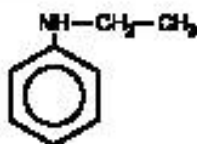
Рисунок В.7 — Молекулярная структура Н-этилфениламина
