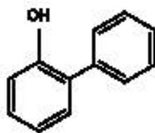
Рисунок В.9 — Молекулярная структура ортофенилфенола
