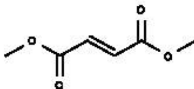
Рисунок В.4 — Молекулярная структура диметилфумарата
