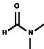
Рисунок В.3 — Молекулярная структура ДМФА
