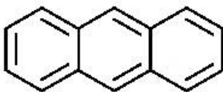
Рисунок В.17 — Структура антрацена
