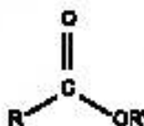
Рисунок A.2 — Эфирная связь
