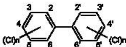
Рисунок В.13 — Молекулярная структура ПХБФ
