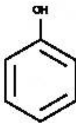
Рисунок В.18 — Структура фенола
