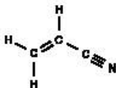
Рисунок В.1 — Молекулярная структура акрилонитрила
