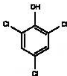
Рисунок В.14 — Молекулярная структура и номер по CAS полихлорфенолов
