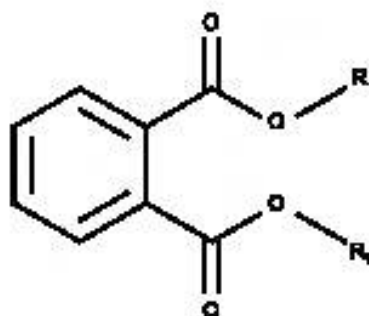
Рисунок В.12 — Молекулярная структура фталатов
