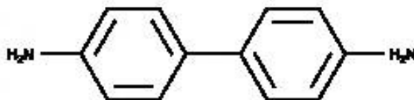
Рисунок В.2 — Пример молекулярной структуры ароматических аминов. Бензидин
