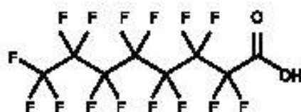
Рисунок В.11 — Молекулярная структура ПФОК
