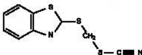
Рисунок В.15 — Молекулярная структура ТЦМТБ
