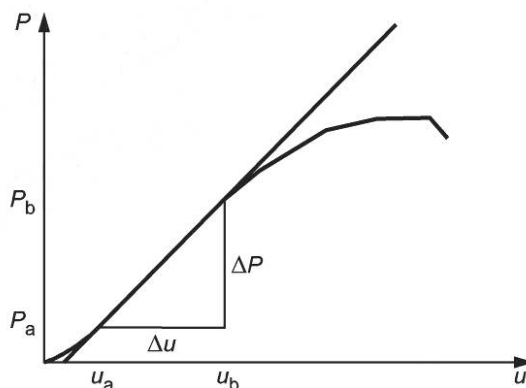
Рисунок 2 — График зависимости нагрузки от перемещения пластин
