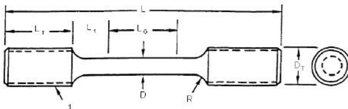
Рисунок 2 — Образец с резьбовой зажимной частью
