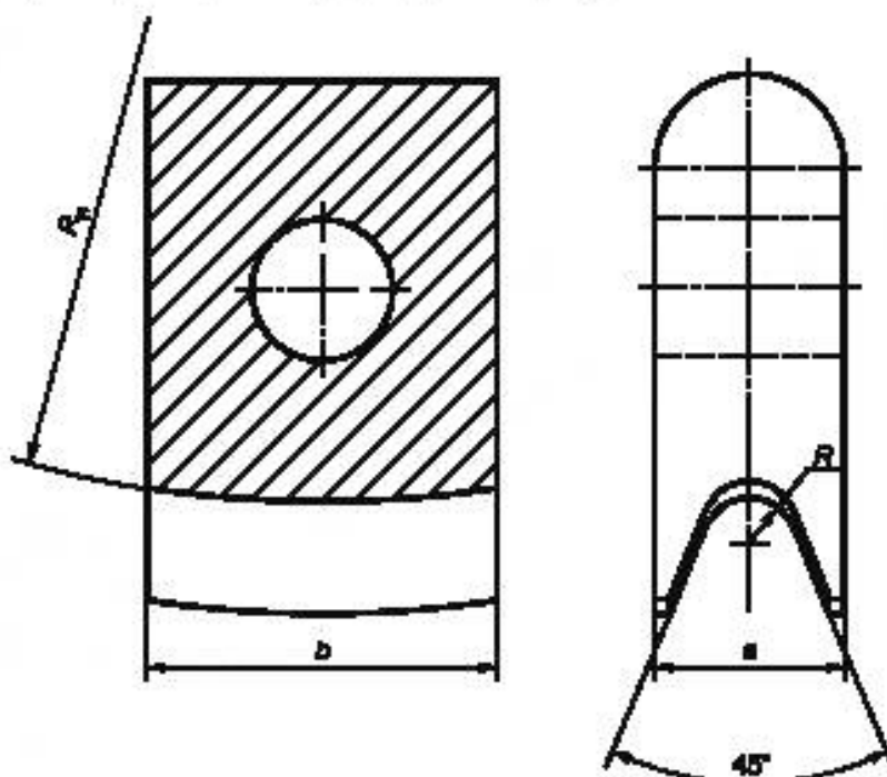
Рисунок 1 — Пуансон для испытания образцов круглого сечения
