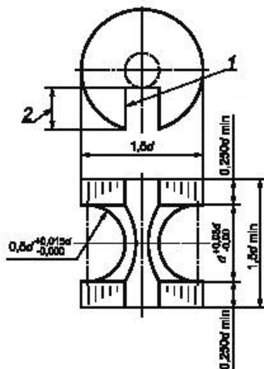
Рисунок 2 — Геометрические размеры опор
