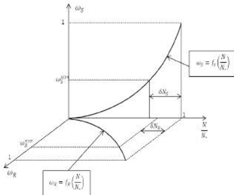
Рисунок 4 — Определение относительного остаточного ресурса
