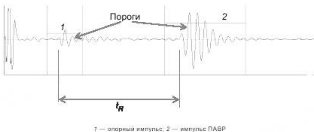
Рисунок 2 — Типичная осциллограмма при измерении преобразователем ПАВР
