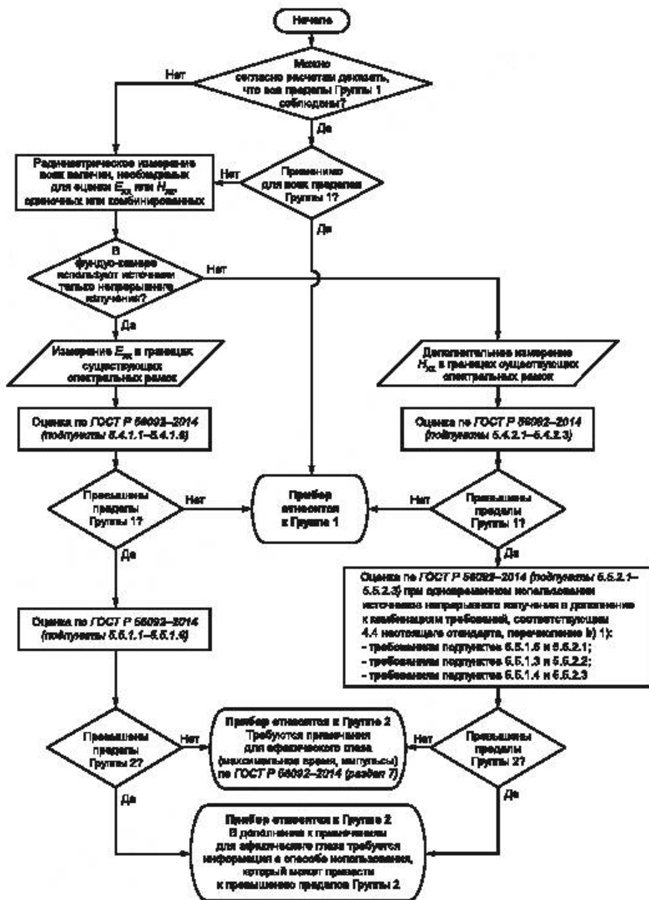
Рисунок А.1 — Блок-схема процедуры
