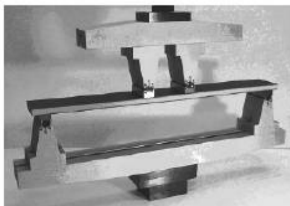
Рисунок 3 — Стандартная схема нагружения в четырех точках
