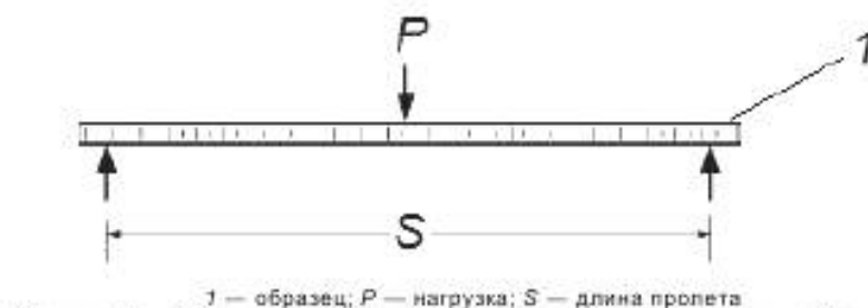
Рисунок 2 — Схема приложения нагрузки при трехточечном изгибе
