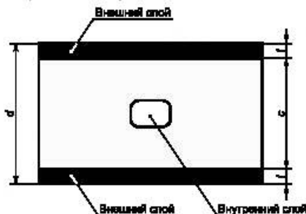
Рисунок 6 — Размеры толщин «сэндвич»-конструкции
