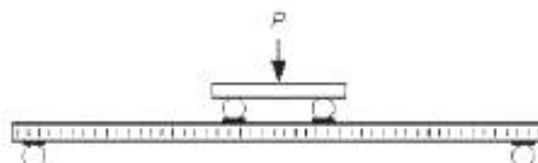
Рисунок 1 — Испытываемый образец и приспособление для проведения испытания
