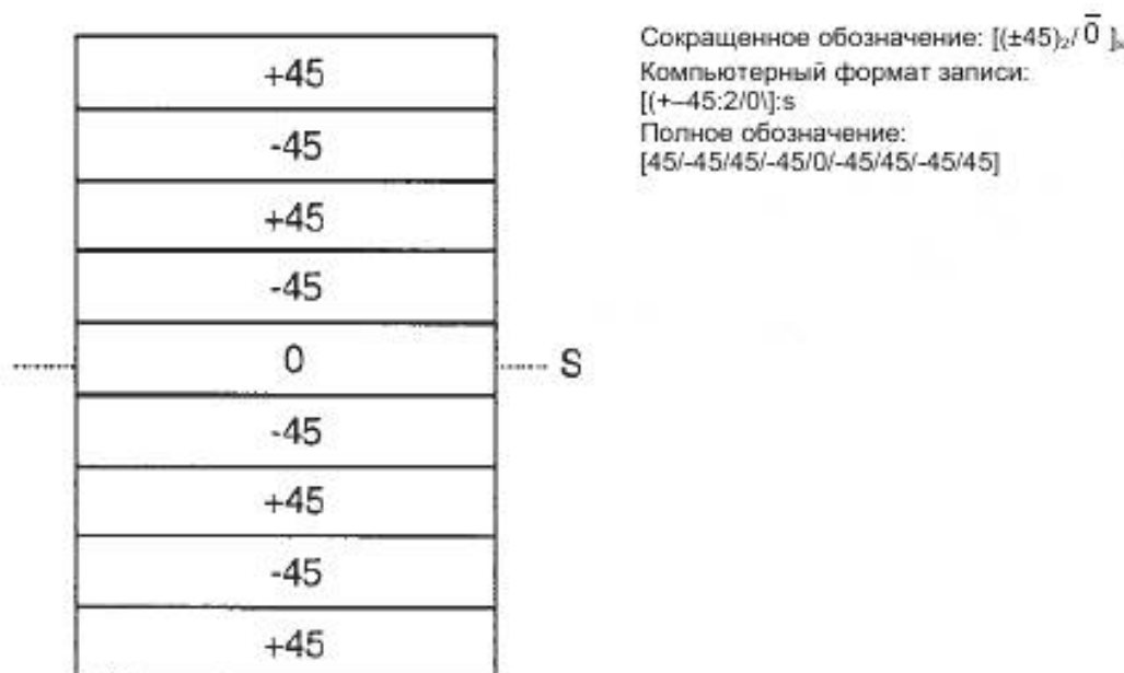
Рисунок 1 – Примеры обозначений направлений армирования
