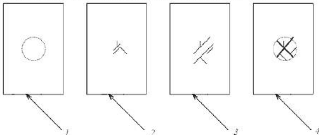
Рисунок А.1 — Внешние типы разрушений
