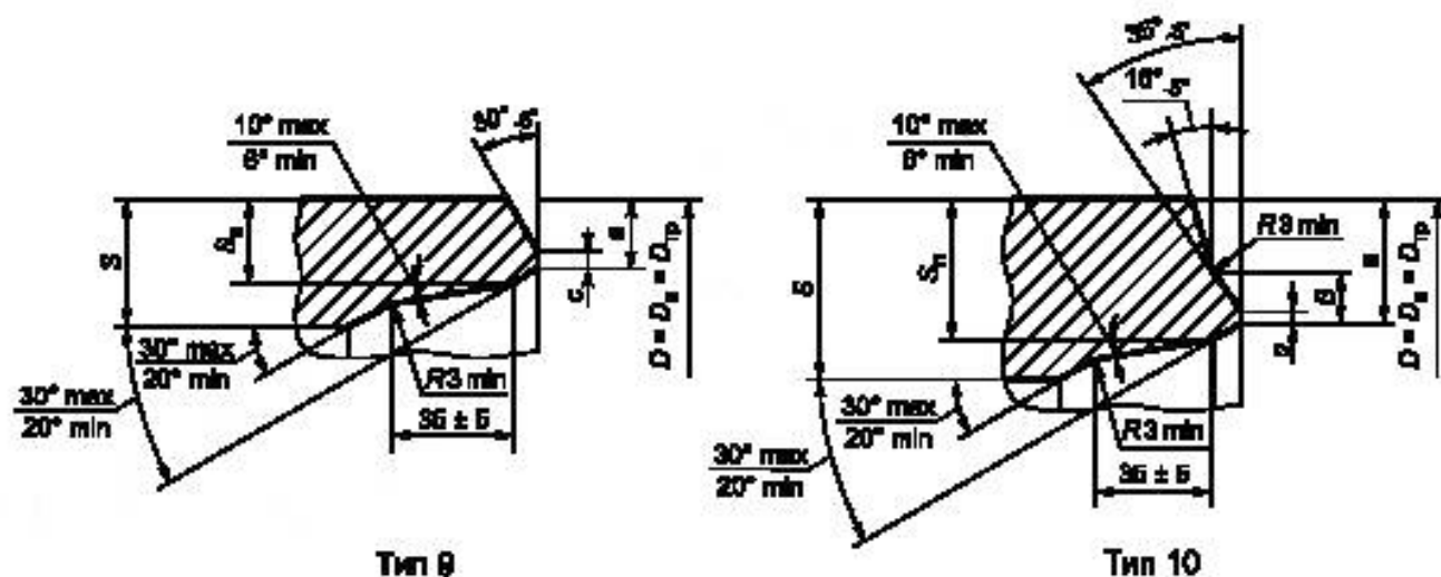
Рисунок 3, лист 2 — Типы разделки кромок торцов детали
