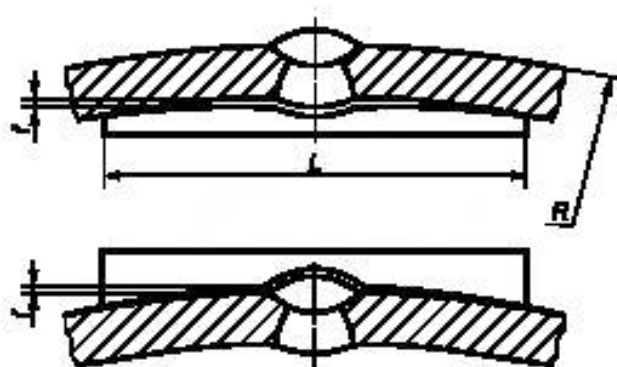
f — максимальный зазор между шаблоном и поверхностью детали; R — номинальный наружный радиус детали; L — длина шаблона
