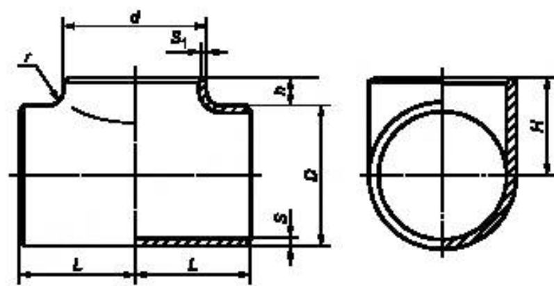
а) равнопроходной тройник
