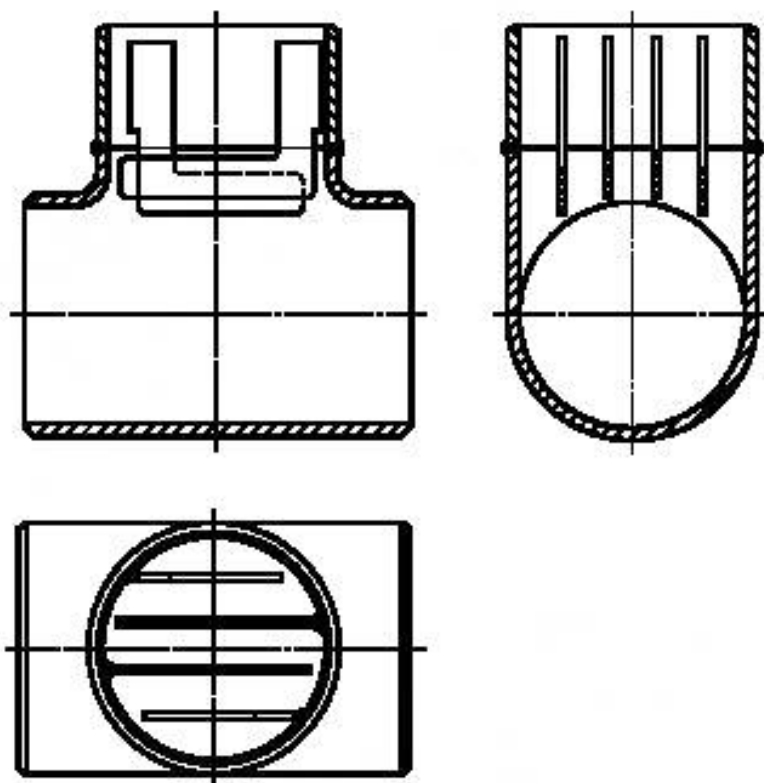
Рисунок А.1 — Решетка тройника
