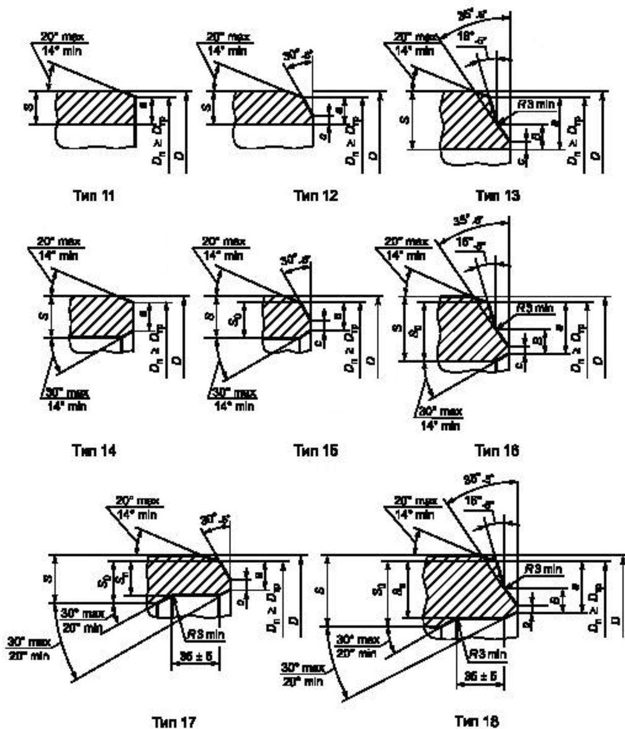
Рисунок 3, лист 3 — Типы разделки кромок торцов детали
