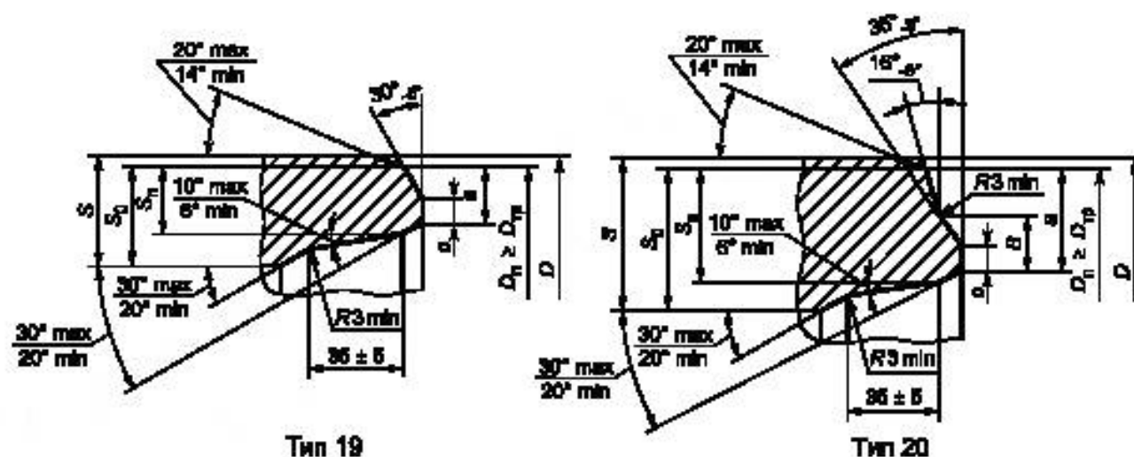
Рисунок 3, лист 4 — Типы разделки кромок торцов детали
