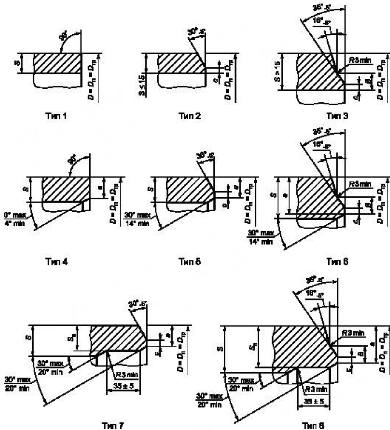
Рисунок 3, лист 1 — Типы разделки кромок торцов детали
