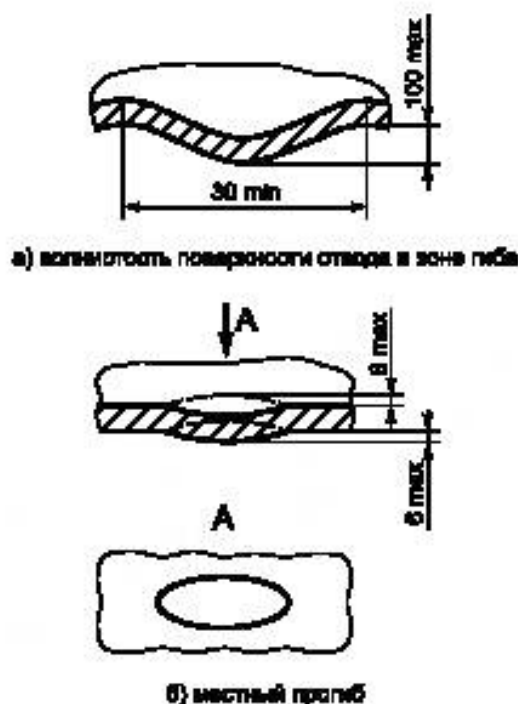
Рисунок 7 — Дефекты формы ОГ
