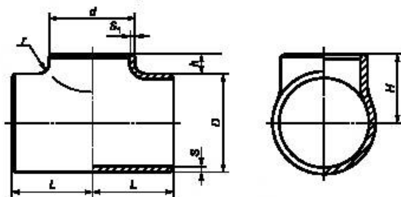
б) переходный тройник
