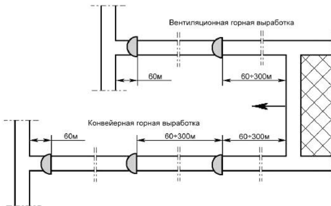
Рисунок В.3 — Схема расположения сланцевых заслонов на добычном участке очистной выработки
