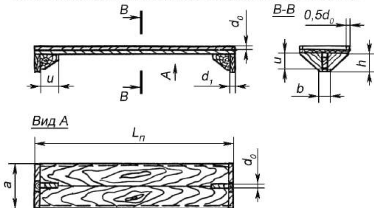
Рисунок 1 — Полка сланцевого заслона жесткой конструкции
