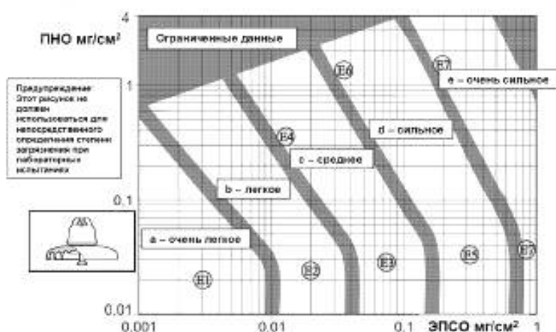
Рисунок 1 — Определение областей классов степени загрязнения в эксплуатации (СЗЗ) типа А по зависимостям плотности нерастворимых осадений (ПНО) от эквивалентной плотности солевых отложений (ЭПСО) для стандартного тарельчатого изолятора
