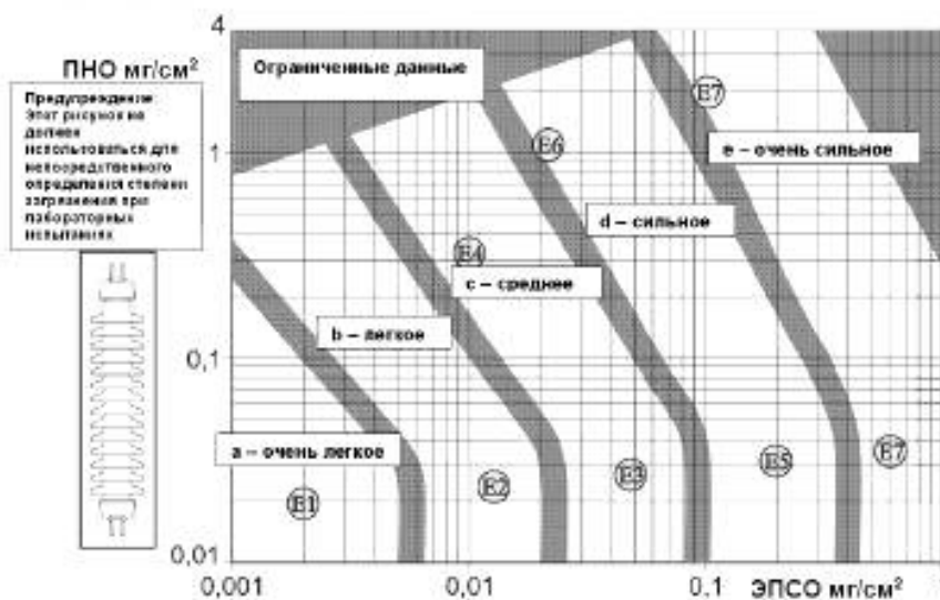
Рисунок 2 — Определение областей классов степени загрязнения в эксплуатации (СЗЗ) типа А по зависимостям плотности нерастворимых осадений (ПНО) от эквивалентной плотности солевых отложений (ЭПСО) для стандартного длинностержневого изолятора
