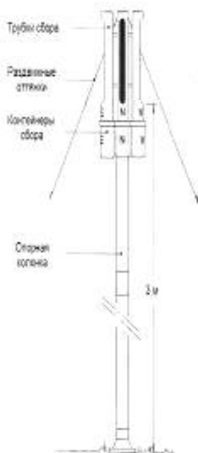
Рисунок Е.1а — Общий вид устройства
