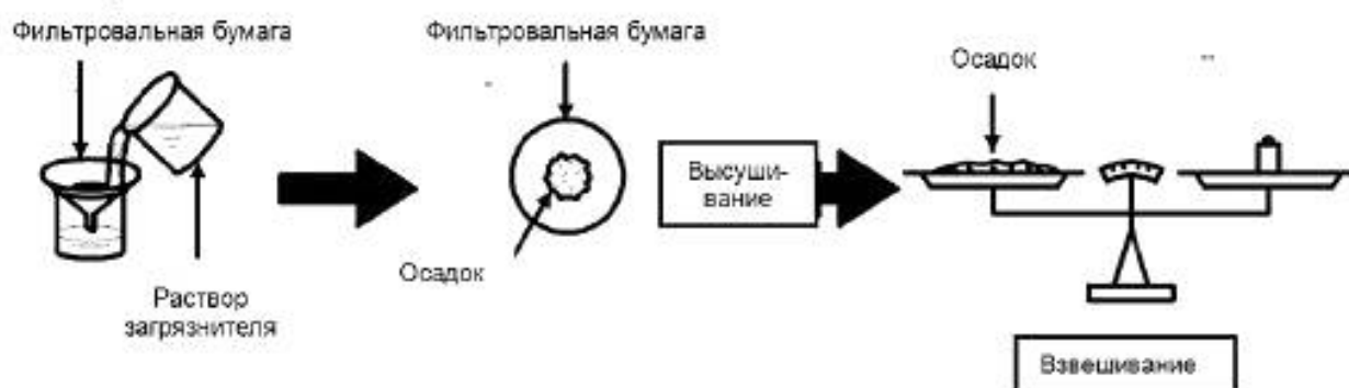
Рисунок С.5 — Методика измерения ПНО
