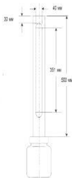
Рисунок Е.1б — Размеры прорези
