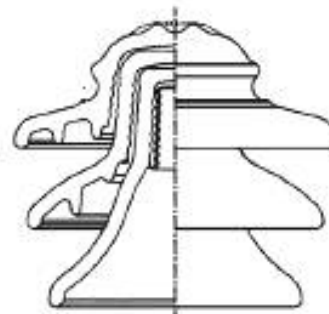
Рисунок 6б — Многоэлементный штыревой изолятор
