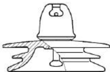
Рисунок 5а — Тарельчатые изоляторы с переменным вылетом ребра
