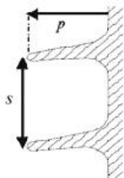
Рисунок 8а — Постоянный вылет ребер
