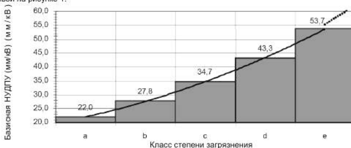
Рисунок 1 — БНУДПУ в функции от класса СЗЭ
