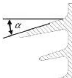
Рисунок 14а — Измерение угла наклона ребра \alpha (измеряется в средней точке)
