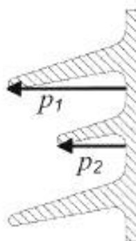
Рисунок 7 — Переменный профиль ребер
