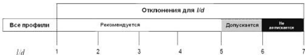
Рисунок 13 — Рекомендации по выбору оптимального соотношения длины пути утечки к межреберному расстоянию
