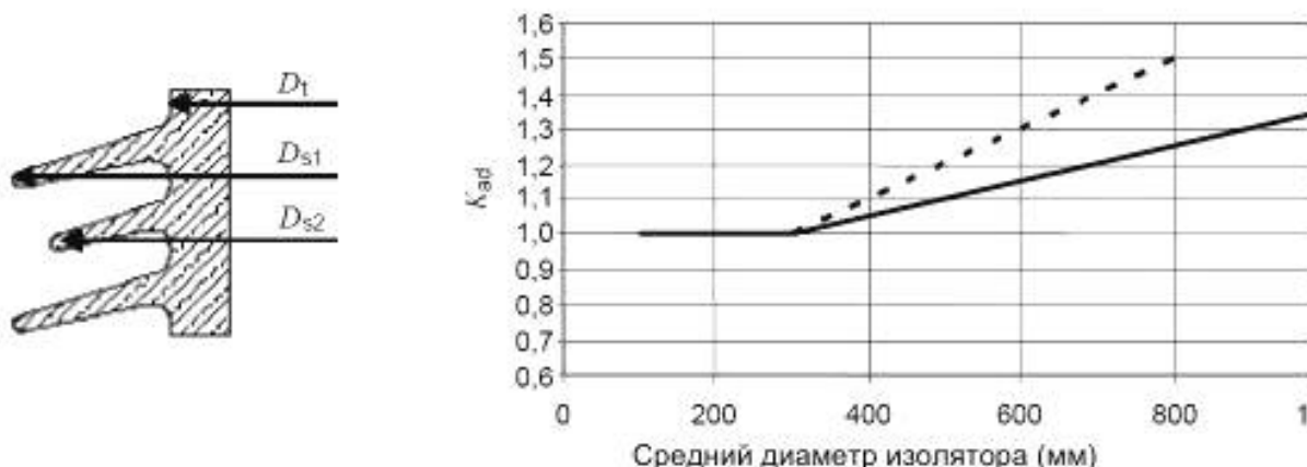
Рисунок 16 — K_{ad} в зависимости от диаметра изолятора
