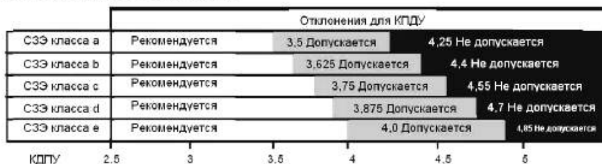
Рисунок 15 — Рекомендации по выбору коэффициента длины пути утечки
