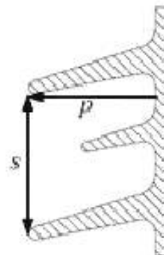
Рисунок 8б — Переменный вылет ребер
