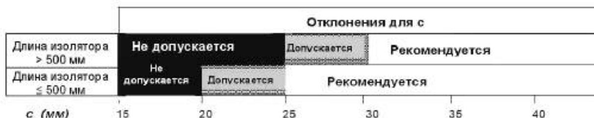
Рисунок 11 — Рекомендации по выбору межреберного расстояния
