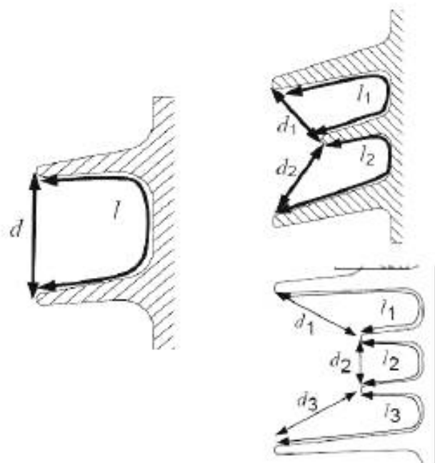
Простой профиль ребра
