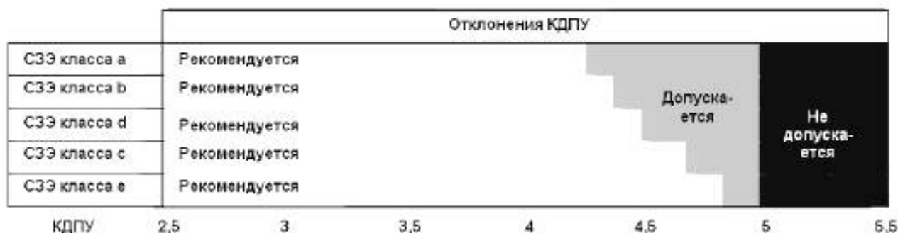
Рисунок 16 — Рекомендации по выбору коэффициента длины пути утечки
