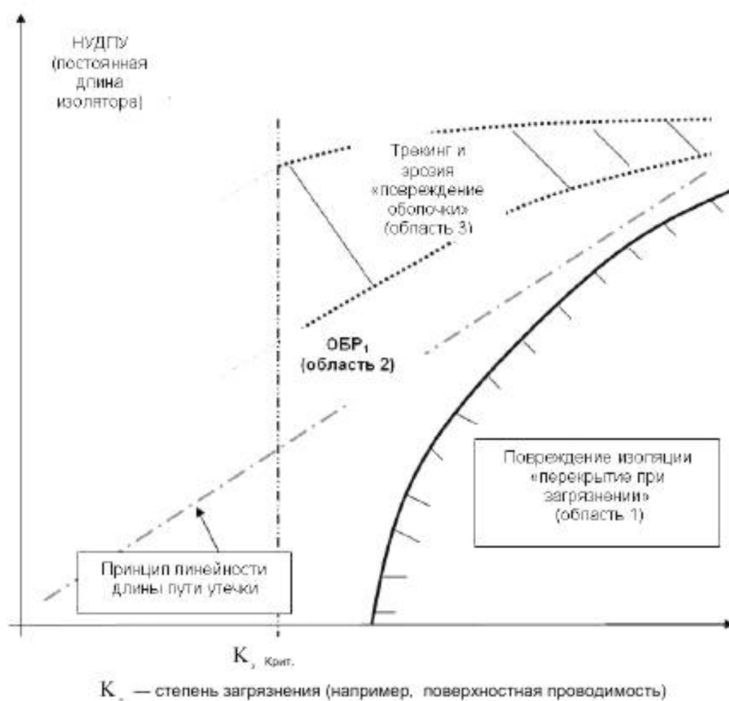
Рисунок А.1 — Области работы в функции от степени загрязнения и НУДПУ (для фиксированной длины изолятора)
