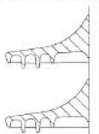
Рисунок 5 — Типичный профиль с глубокими канавками под ребром
