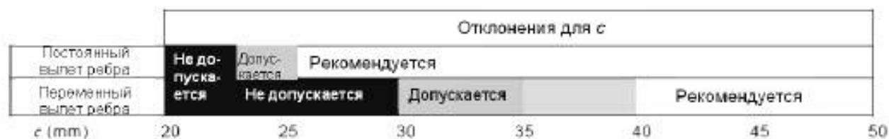
Рисунок 11 — Рекомендации по выбору межреберного расстояния
