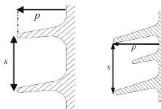
Постоянный вылет ребра
