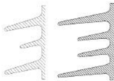
Рисунок 6 — Типичный профиль с переменным вылетом ребра
