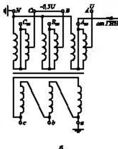
Рисунок DA.2.6 — Пофазное испытание трехобмоточного автотрансформатора
