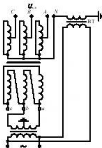
Рисунок ДА.3.5 — Испытание фазы В с подпорным напряжением в нейтрали
