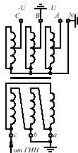
Рисунок DA.2.5 — Одновременное испытание изоляции относительно земли крайних фаз А и С трансформатора
