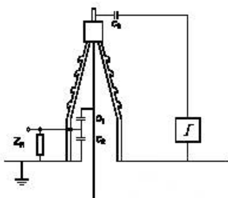
Рисунок А.1 — Схема для калибровки измерения интенсивности частичных разрядов с использованием измерительного вывода конденсаторного типа
