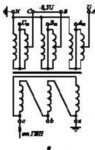
Рисунок DA.2.6 — Пофазное испытание трехобмоточного автотрансформатора
