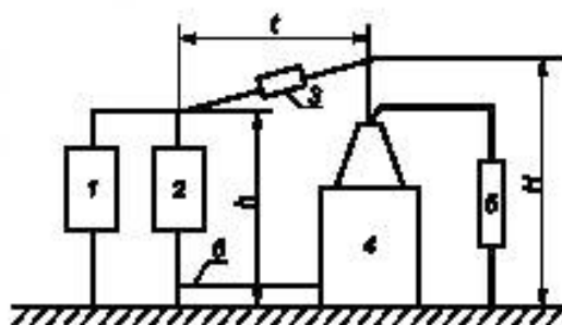
1 — генератор импульсных напряжений; 2 — срез; 3 — демпфирующее сопротивление; 4 — испытуемый объект; 5 — измерительное устройство (делитель напряжения); 6 — провод, соединяющий заземленный бак с заземлением срезом
