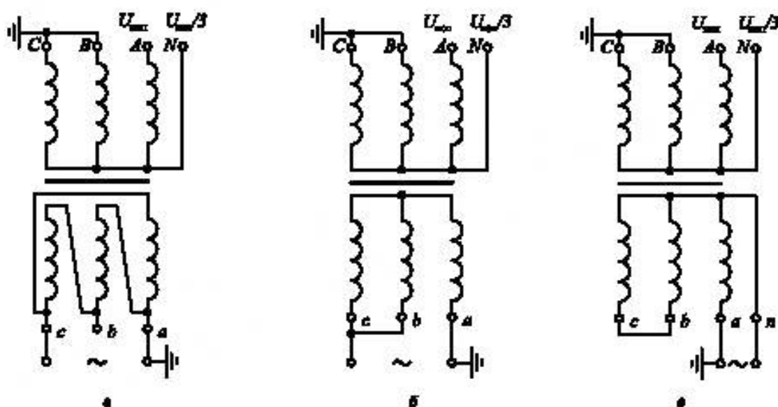
Рисунок ДА.3.1 — Пофазное испытание трехфазного трансформатора
