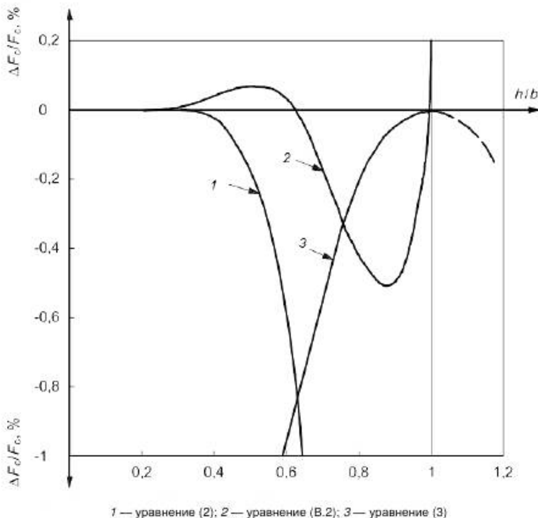
Рисунок В.1 — Относительная погрешность \Delta F_c/F_c при расчете размерного поправочного коэффициента F_c при помощи приближенных уравнений (2), (3) и (В.2) по сравнению с точным уравнением (В.1)
