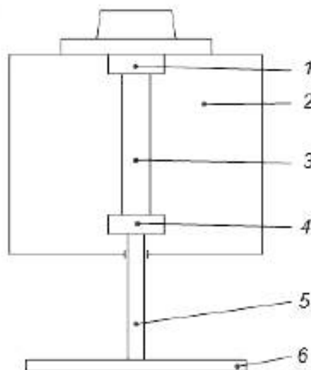
1 — верхний (неподвижный) зажим; 2 — температурная камера; 3 — образец для испытания; 4 — нижний (подвижный) зажим; 5 — стержень; 6 — инерционная деталь
