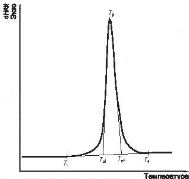
Рисунок 1 — Кривая ДСК с экзотермическим пиком (метод сканирования по температуре)
