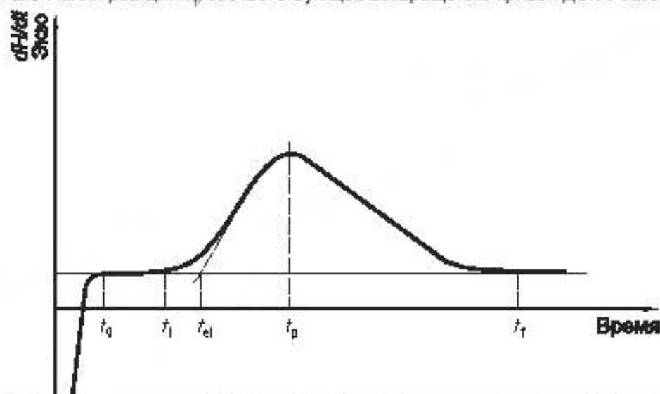
Рисунок 2 — Кривая ДСК с экзотермическим пиком (изотермический метод)
