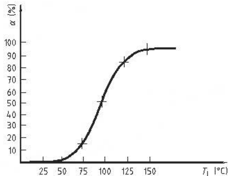
Рисунок 5 — Пример увеличения \alpha с температурой
