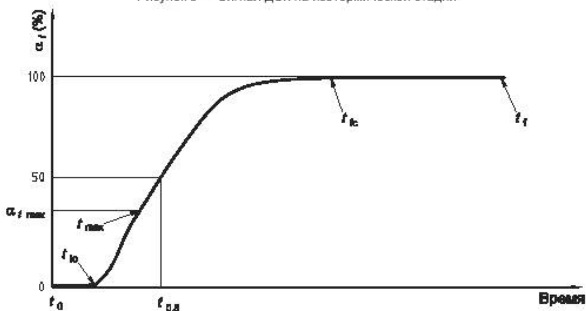
Рисунок 4 — Изменение \alpha_t на изотермической стадии
