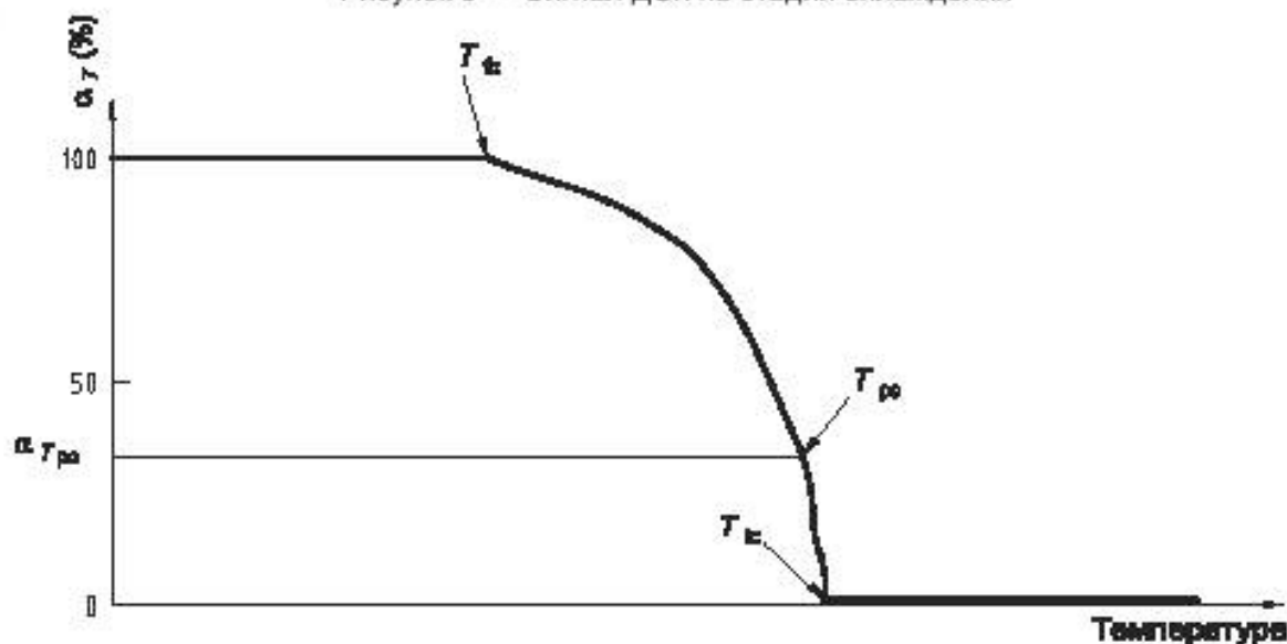
Рисунок 6 — Изменение \alpha_T на стадии охлаждения
