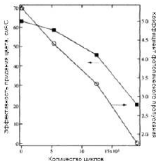
Рисунок 6 — Коэффициент фотооптического пропускания и эффективность придания цвета в виде функции количества циклов применительно к типовому окну с ЭХП
