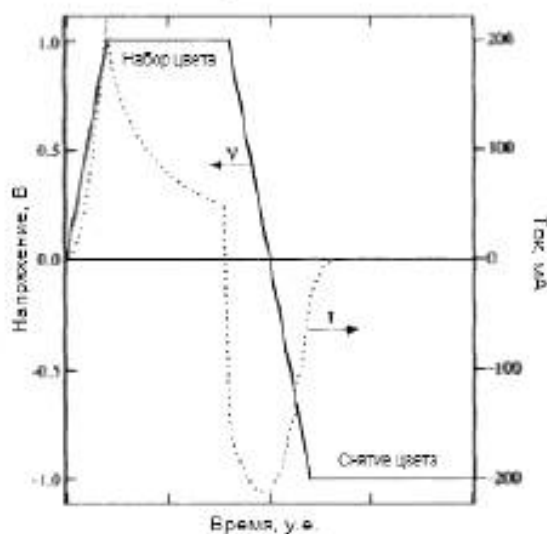
Рисунок 3 — Зависимость напряжения от тока в качестве функции времени в течение набора и снятия цвета у типовых окон с ЭХП
