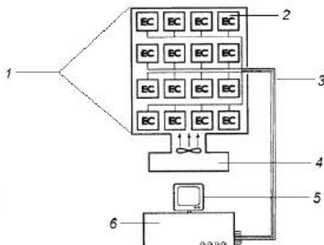
1 — плоскость испытания 1220 × 1830 мм; 2 — стекла с ЭХП; 3 — электрические выводы и кабели термпар; 4 — термошкаф; 5 — компьютер; 6 — многоканальная цифровая автоматизированная система управления и сбора данных
