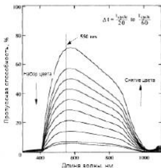
Рисунок 4 — Типовые спектры пропускания
