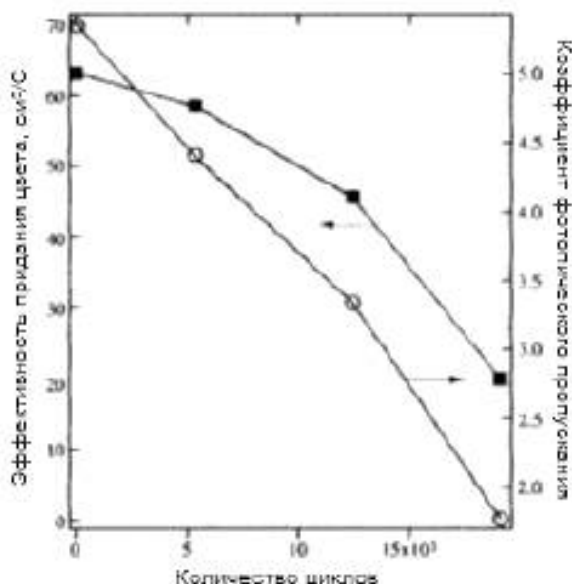
Рисунок 6 — Коэффициент фотопического пропускания и эффективность придания цвета в виде функции количества циклов применительно к типовому окну с ЭХП
