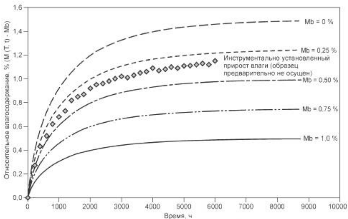
Рисунок А.3.1 — Прогноз влагосодержания для различных уровней начального содержания влаги
