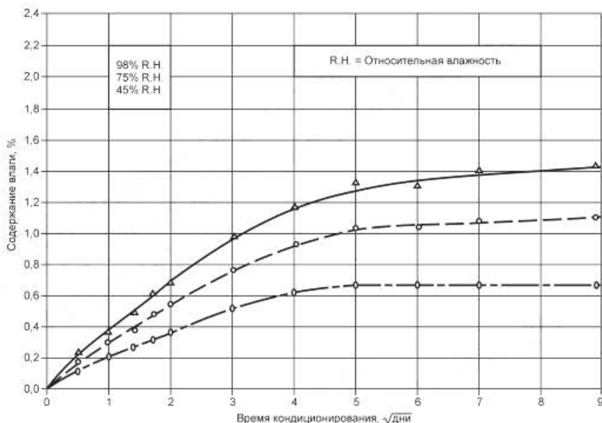
Рисунок 1 — Пример графика влагопоглощения углерод/эпоксидных (0,45—45,0) 2 слоистых материалов из восьми слоев при температуре 48,9 °C (8)
