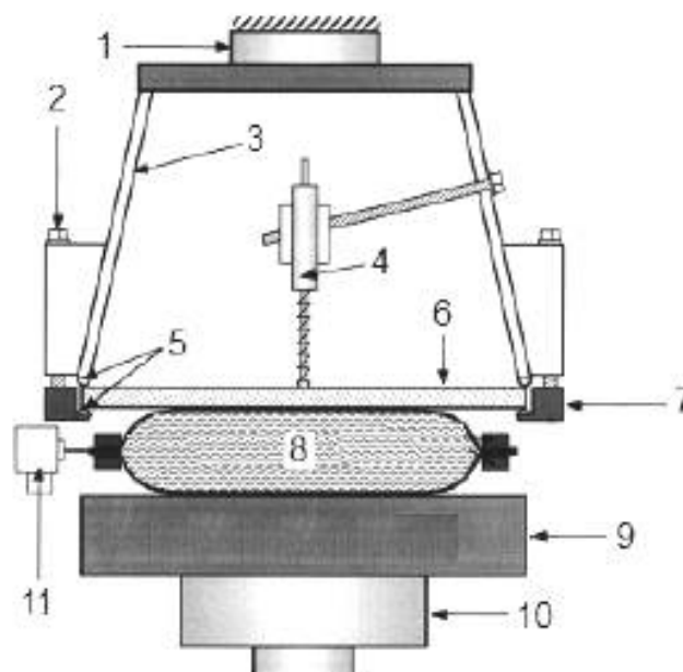
1 — датчик нагрузки; 2 — болты крепления, соединяющие верхнюю и нижнюю части приспособления для испытания; 3 — верхняя часть приспособления для испытания; 4 — датчик перемещения; 5 — опорные подшипники; 6 — образец; 7 — нижняя часть приспособления для испытания; 8 — эластичный баллон; 9 — опорная плита под эластичный баллон; 10 — подвижная траверса испытательной машины; 11 — манометр
