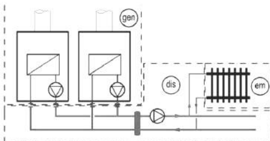
Рисунок 5 — Пример границ подсистем (3)
