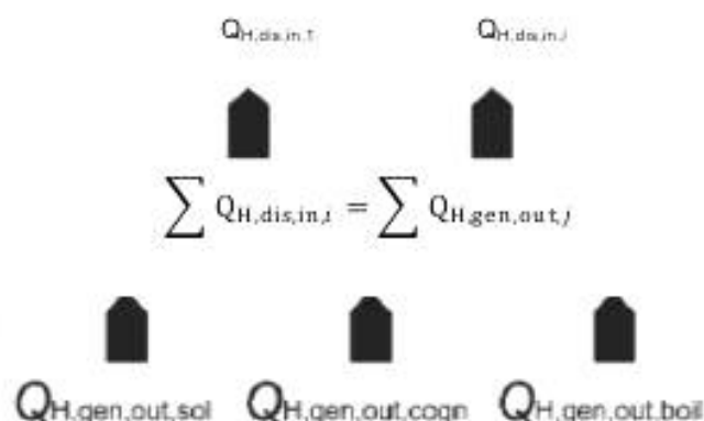
Рисунок 2 — Пример разделения нагрузки между подсистемами теплогенерации
