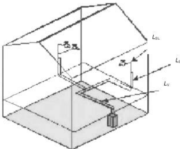
Рисунок Г.1 — Расположение трубопроводов
