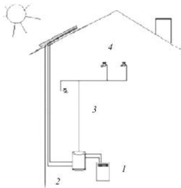
Рисунок 1 — Основные компоненты системы бытового горячего водоснабжения
