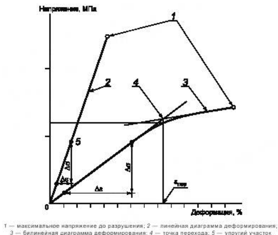
Рисунок 1 — Диаграммы деформирования ПКМ
