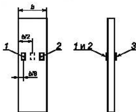
b — ширина образца; 1, 2, 3 — датчики
