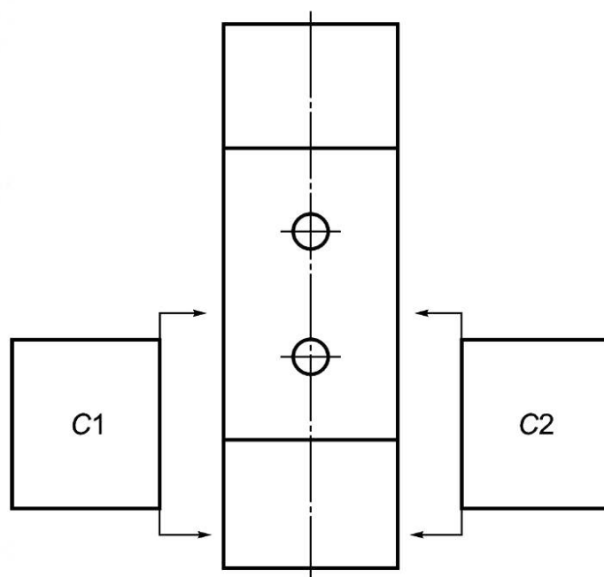
Рисунок 5 — Установка датчиков деформации на боковых сторонах образца
