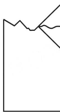
Рисунок В.8 — Разрушение при растяжении типа MGM: многотиповое разрушение через центр отверстия (сопровождается деламинацией и разделением на части)
