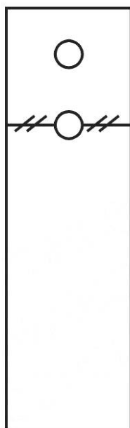
Рисунок В.9 — Разрушение при сжатии типа LGM: поперечное разрушение через центр отверстия (как правило, происходит вдоль направления армирования 0^\circ )
