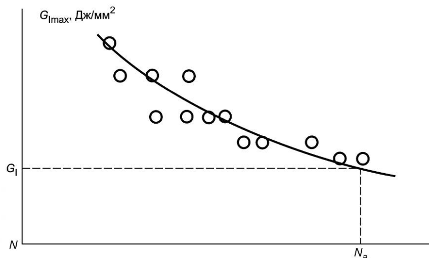
Рисунок 2 — Кривая G—N
