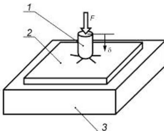
1 — индентор; 2 — образец; 3 — опора; F — контактная нагрузка
