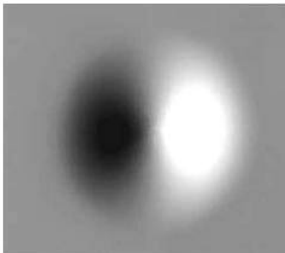
Рисунок 4 — Шерограмма без интерференционных полос
