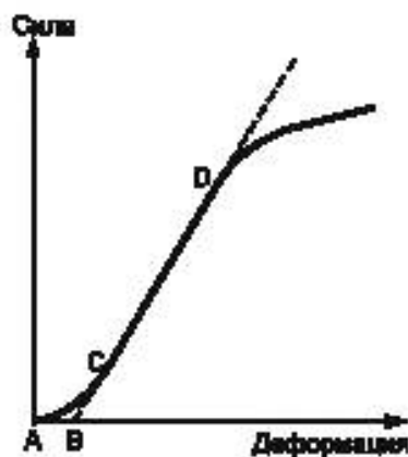
Рисунок А.1 — График зависимости силы от деформации
