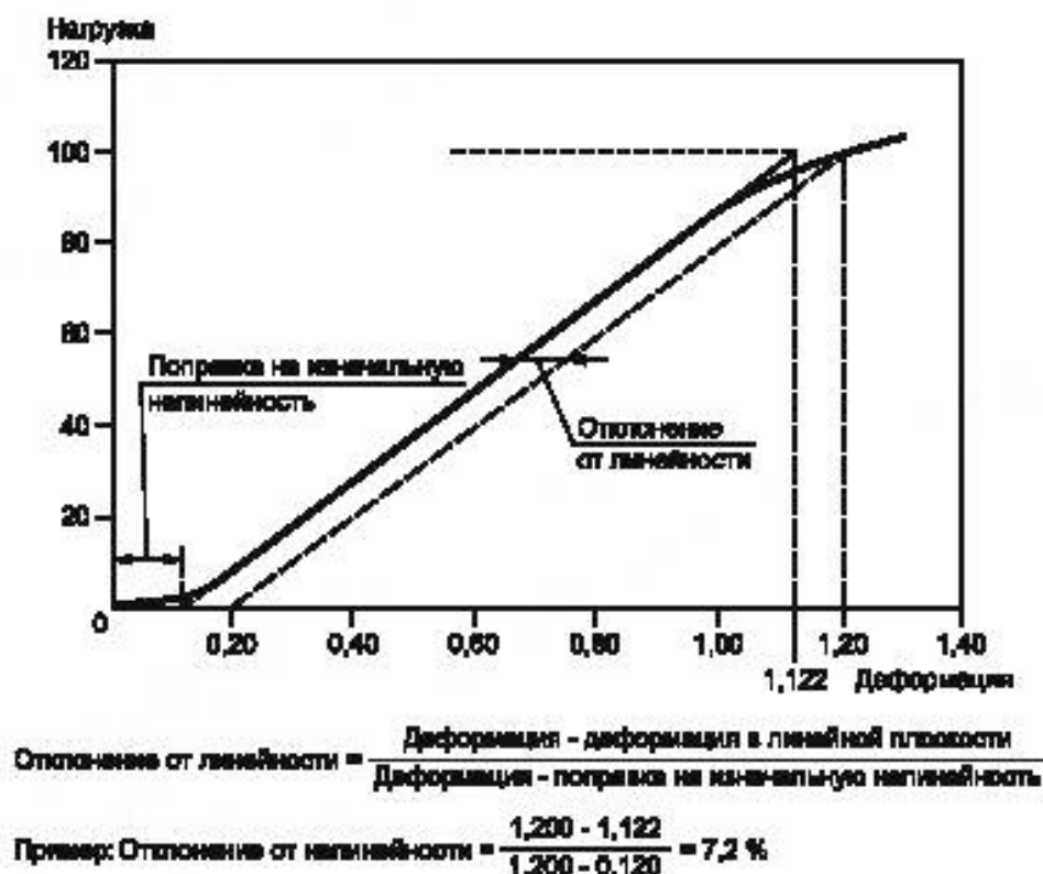
Рисунок 2 — Определение отклонения от линейности
