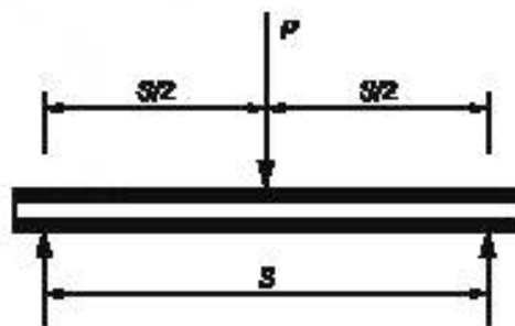
(a) трехточечное нагружение (C393/C393M стандартная схема)
