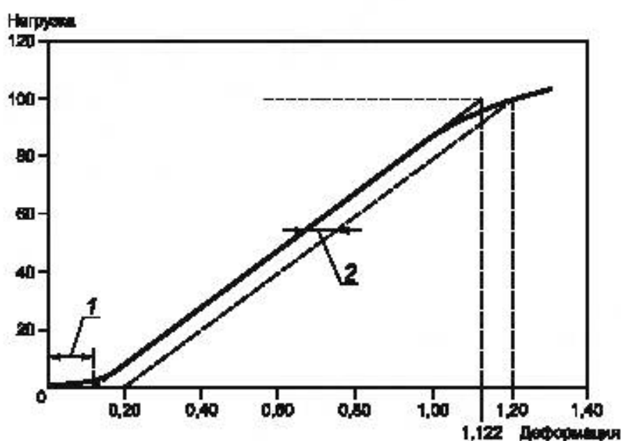
Рисунок 1 — Отклонение от линейности
