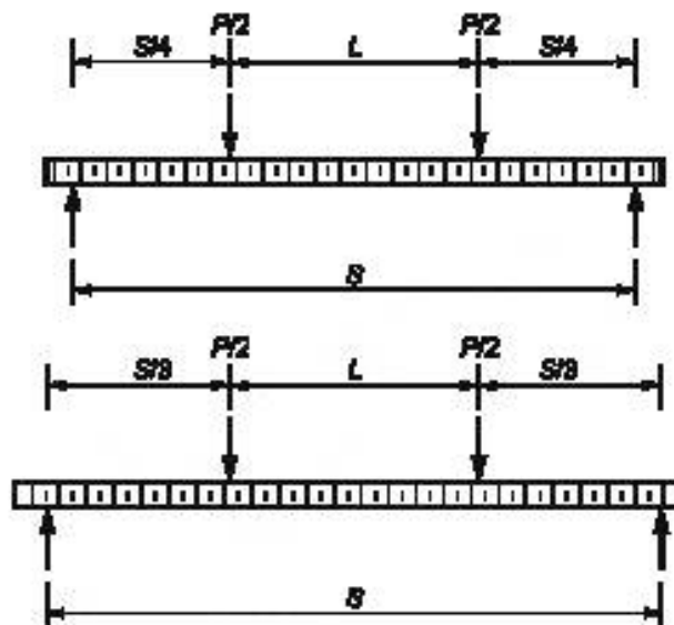
(c) четырехточечное нагружение (C393/C393M нестандартная схема)
