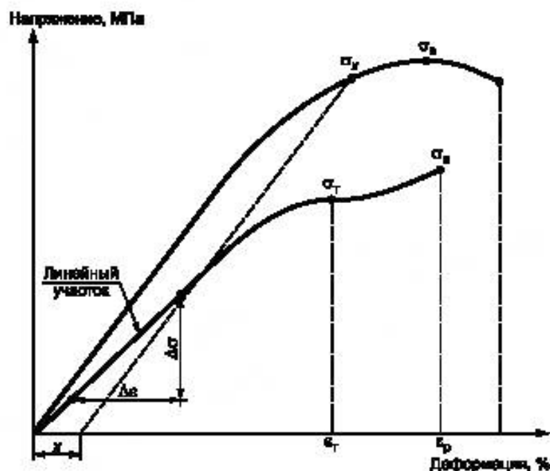
Рисунок 1 — Типовые диаграммы деформирования
