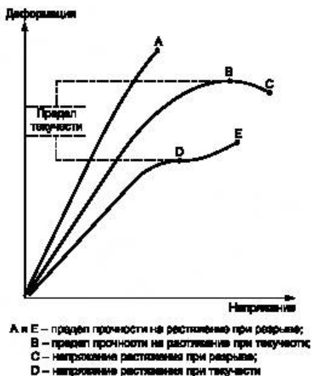
Рисунок A2.3 — Обозначения свойств при растяжении
