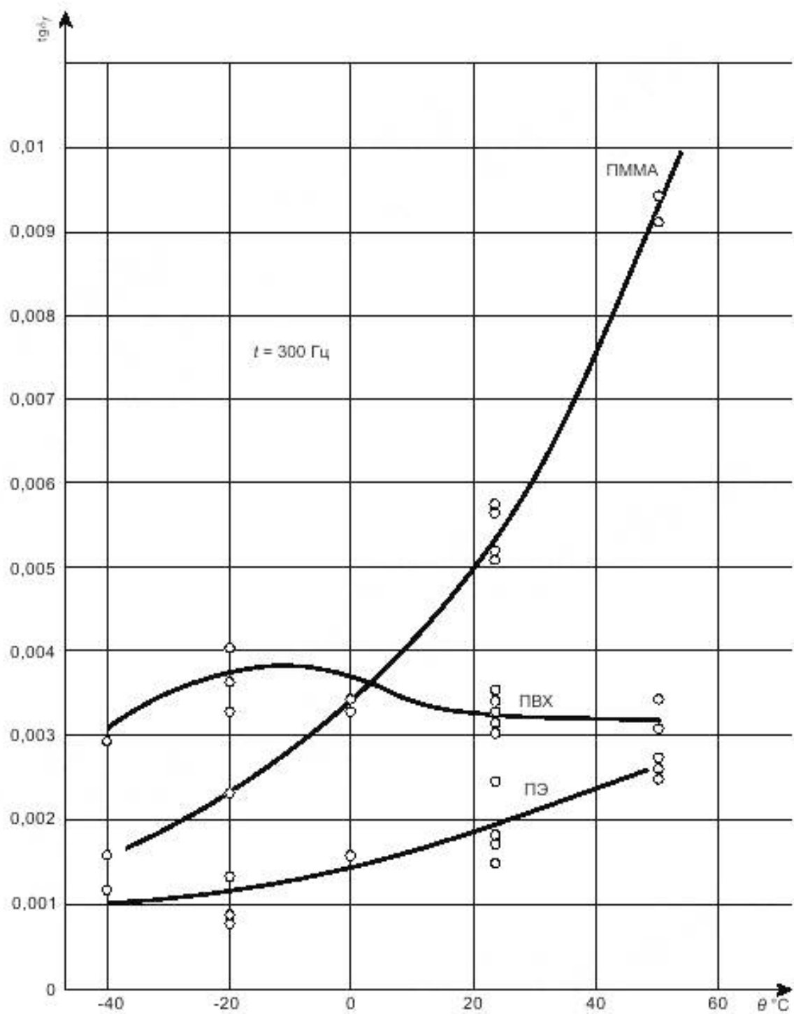
Рисунок А.3 — Тангенс угла механических потерь при изгибе ( \text{tg } \delta_f ) в зависимости от температуры для полиметилметакрилата (ПММА), поливинилхлорида (ПВХ) и полиэтилена (ПЭ), измеренный при частоте 300 Гц
