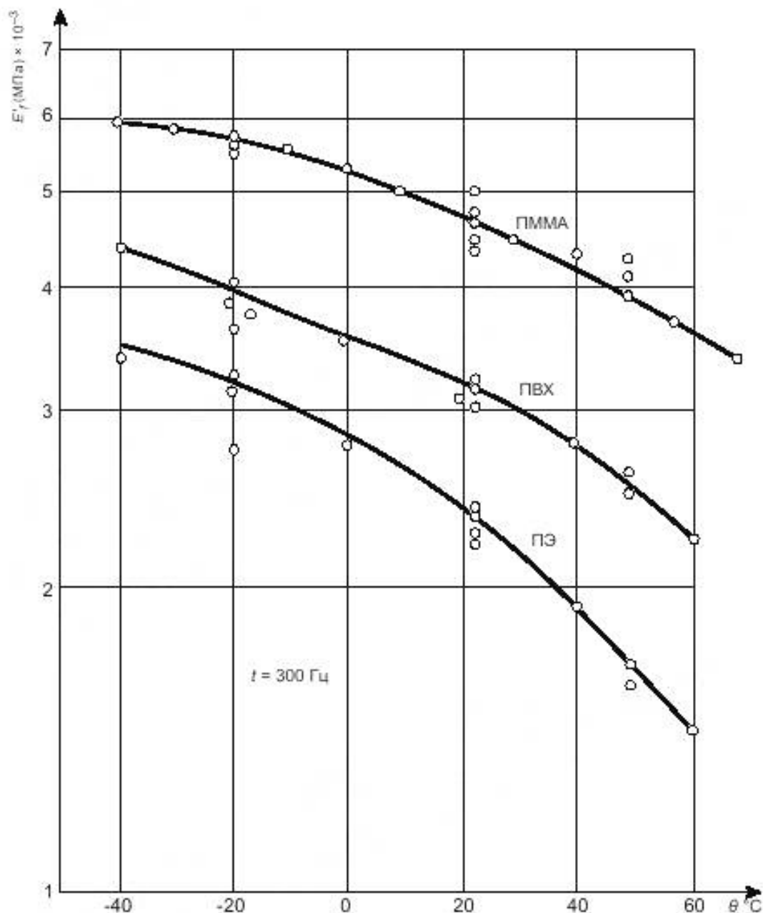
Рисунок А.1 — Действительная часть комплексного модуля при изгибе E' в зависимости от температуры для полиметилметакрилата (ПММА), поливинилхлорида (ПВХ) и полиэтилена (ПЭ), измеренная при частоте 300 Гц
