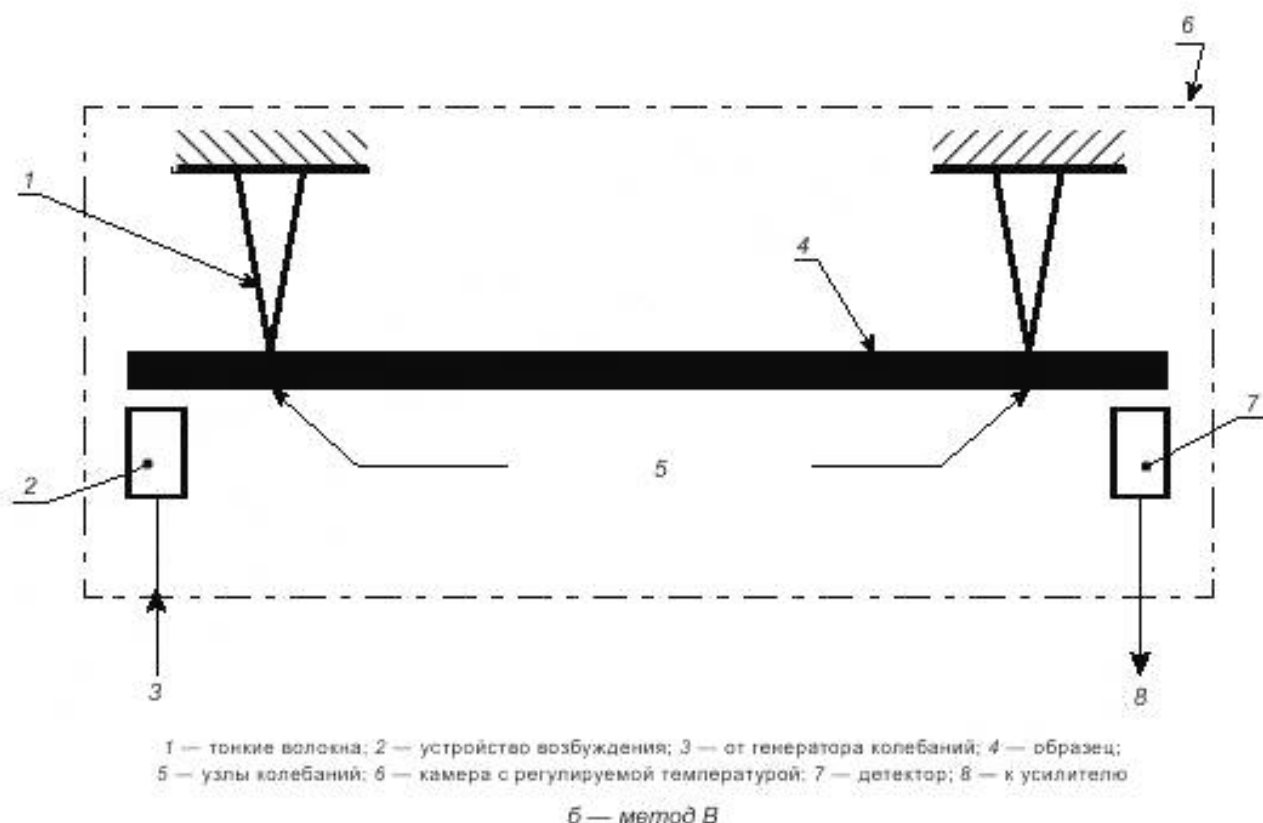
Рисунок 1 — Схематические изображения приборов для проведения испытаний
