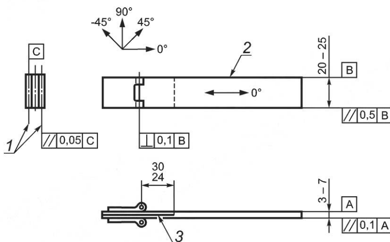
Рисунок 2 — Эскиз образца с начальной межслоевой трещиной
