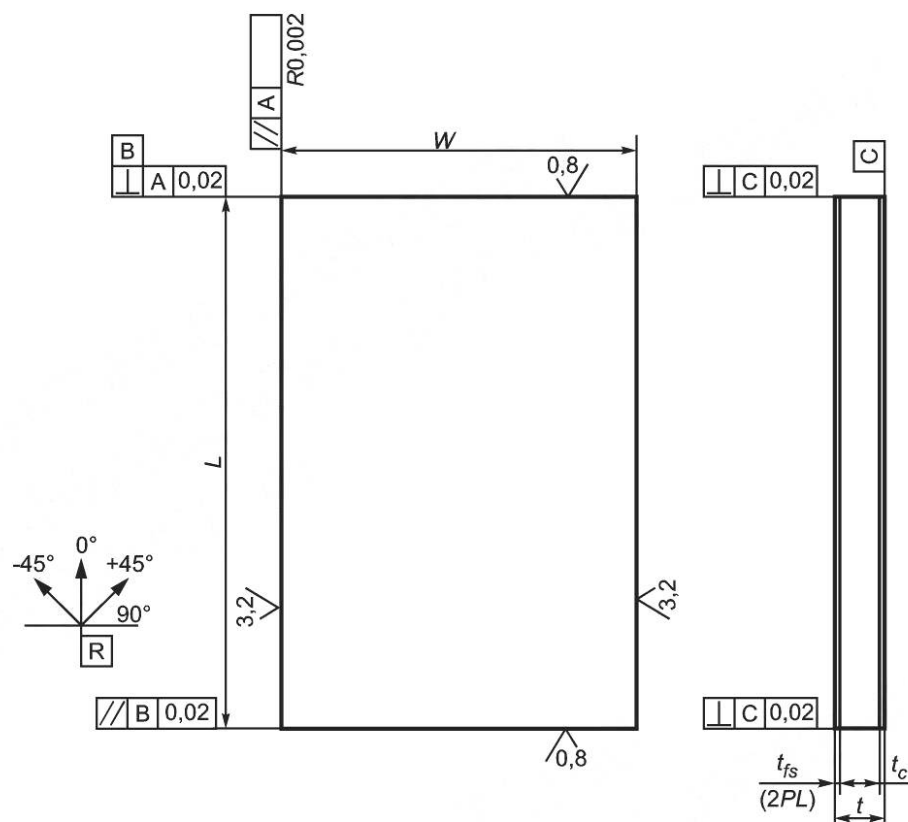
Рисунок 1 — Размеры образцов
