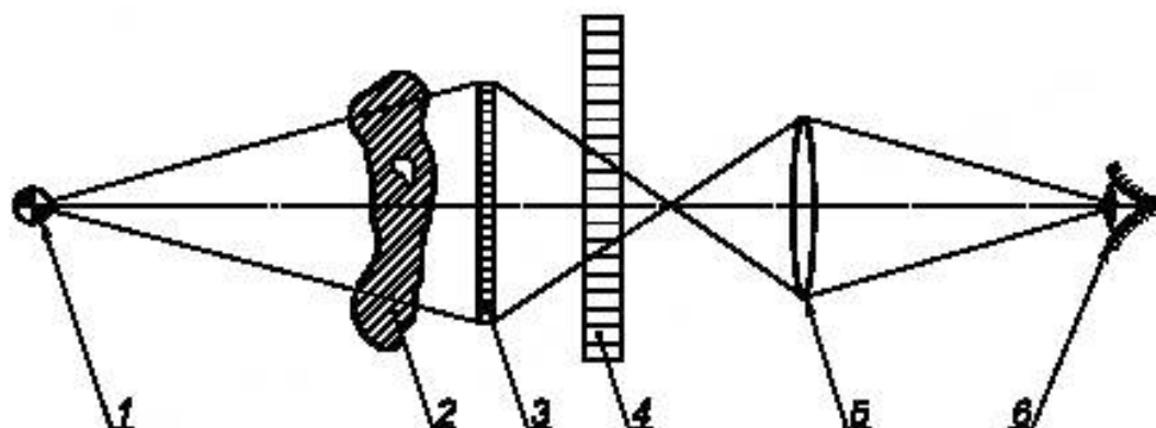
Рисунок ДГ.1 — Основная система радиоскопии
