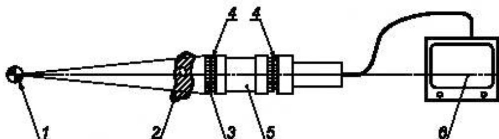
Рисунок ДГ.5 — Система радиоскопии с телевизионной камерой, работающей при низком уровне освещения
