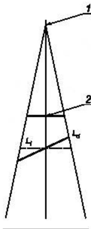
1 — источник излучения; 2 — образец для контроля; L_1 — размер неискаженного изображения; L_2 — размер искаженного изображения
