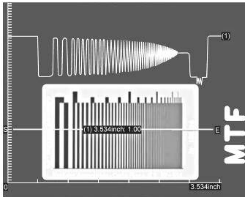
Рисунок ДЕ.6 — Определение разрешения систем формирования изображений
