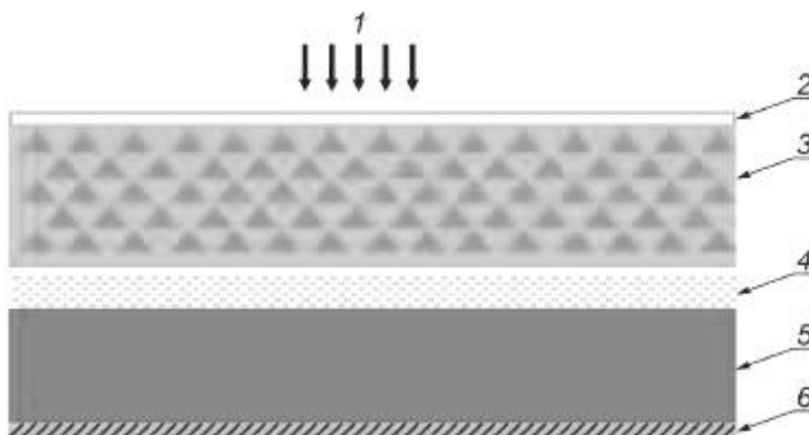
1 — излучение, исходящее из поглощающего материала; 2 — защитный слой; 3 — люминофорный слой (BaF (Cl, Br, I): EU 2+ ); 4 — проводящий слой; 5 — гибкая подложка; 6 — световое экранирование и защитный слой
