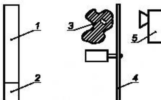
1 — скинциллятор; 2 — фотоумножитель; 3 — образец для контроля; 4 — вращающийся диск с прорезью; 5 — источник рентгеновского излучения
