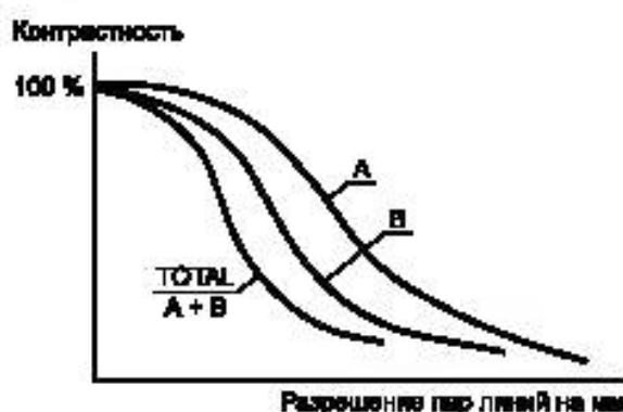
Рисунок ДГ.17 — Типичный график MTF
