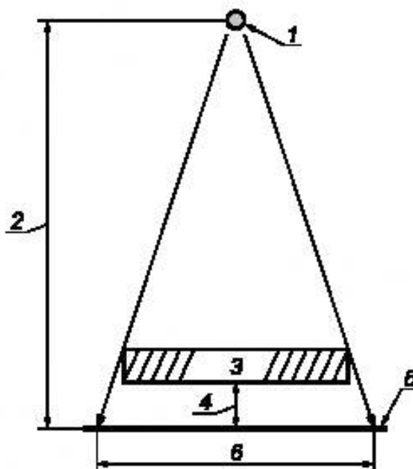
1 — источник излучения; 2 — расстояние от источника до детектора; 3 — образец для контроля; 4 — расстояние от образца для контроля до детектора; 5 — детектор; 6 — оптическое увеличение поля обзора
