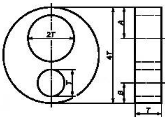
Рисунок 2 — Круглый эталон чувствительности
