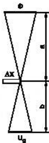
б) Нерезкость, вызванная геометрическими параметрами U_g
