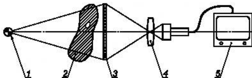
Рисунок ДГ.4 — Система радиоскопии с усилителем света и оптикой
