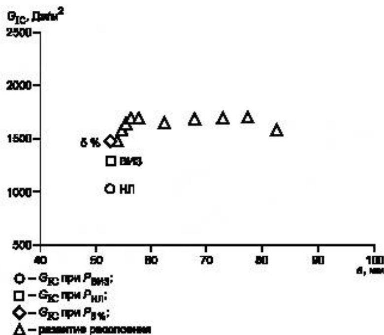
Рисунок 2 — Зависимость вязкости разрушения от длины трещины
