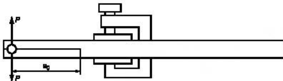
Рисунок 3 — Схема подрачивания трещины перед испытанием
