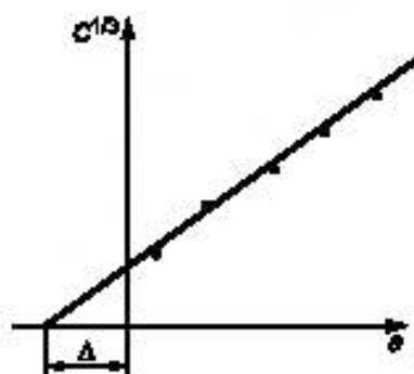
Рисунок 6 — Схема определения поправки |\Delta| к длине трещины
