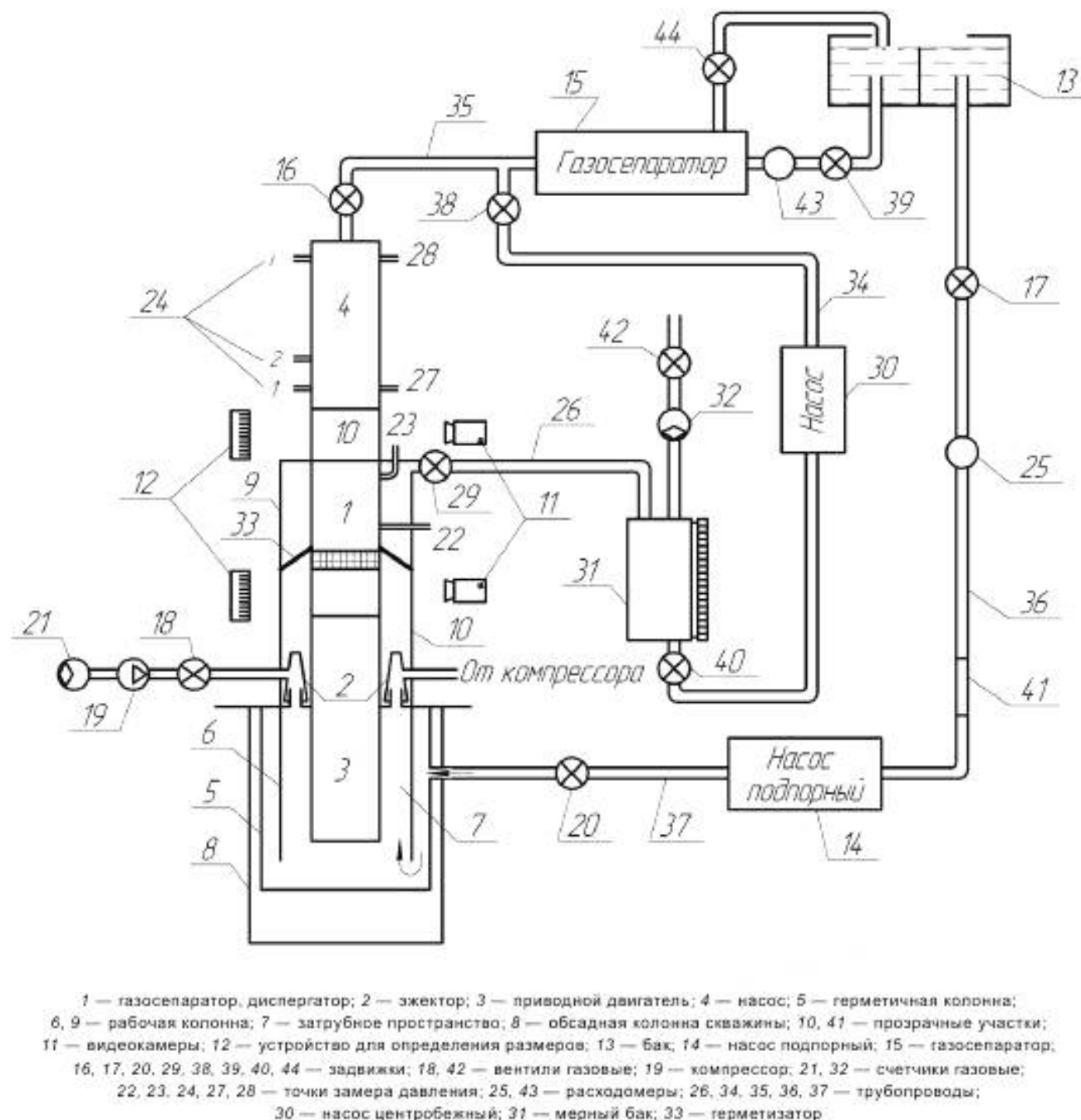
Рисунок Ж.1 — Схема стенда для испытаний газосепараторов и диспергаторов
