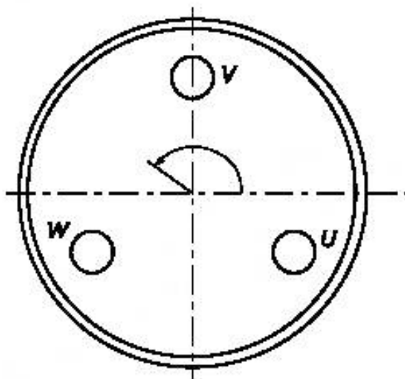
Рисунок Л.1 — Схема расположения нижних выводных концов верхних и средней секций
