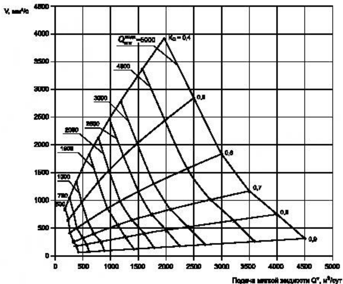
Рисунок А.1 — График изменения оптимальной подачи центробежного и диагонального насоса ( Q_{\text{опт}} = 500 - 5000 м 3 /сут)
