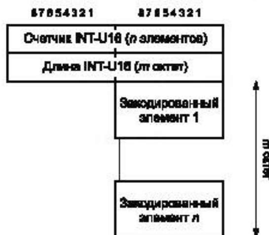
Рисунок A.6 – Кодирование типа SEQUENCE OF
