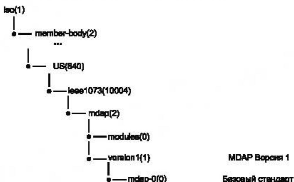
Рисунок В.1 – Присвоение идентификаторов объектов. Корневой путь
