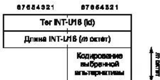
Рисунок А.7 – Кодирование типа CHOICE
