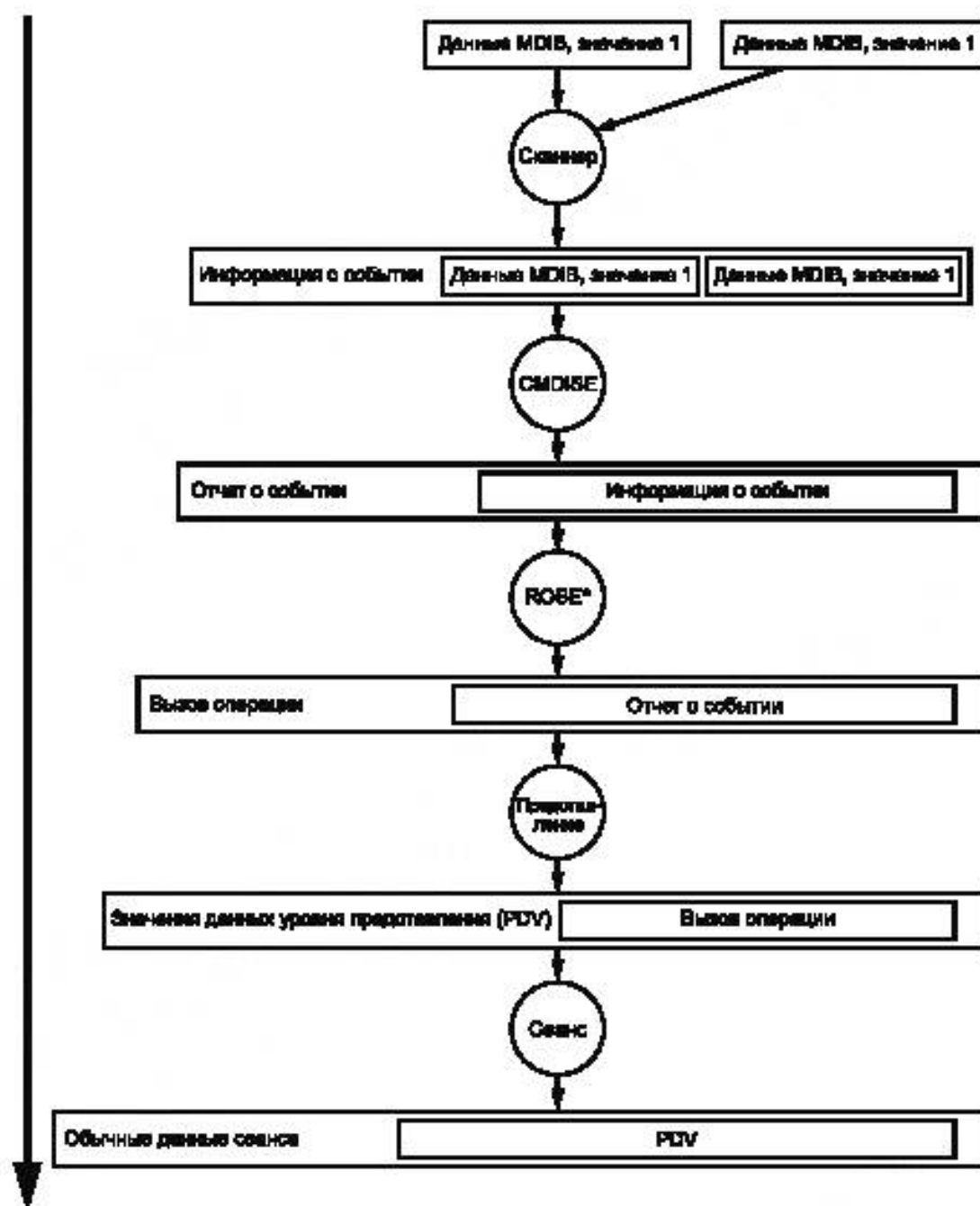
Рисунок 2 — Поток данных, проходящий через коммуникационный стек
