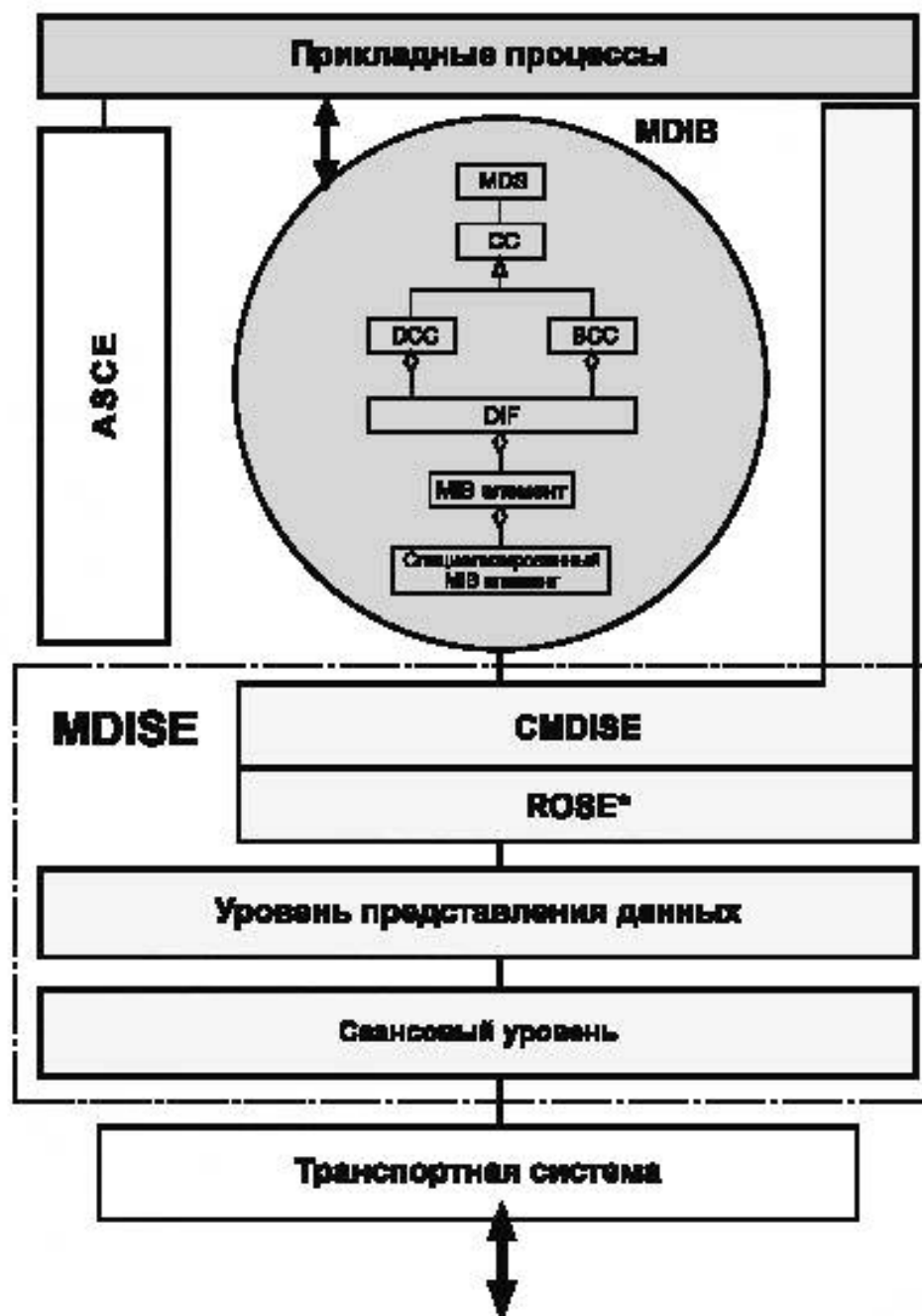
Рисунок 1 – Стек MDC
