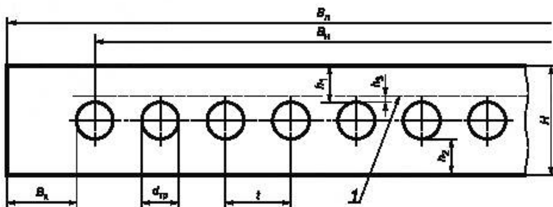
б — С одной защитной тканевой прокладкой (1РТЛ)
