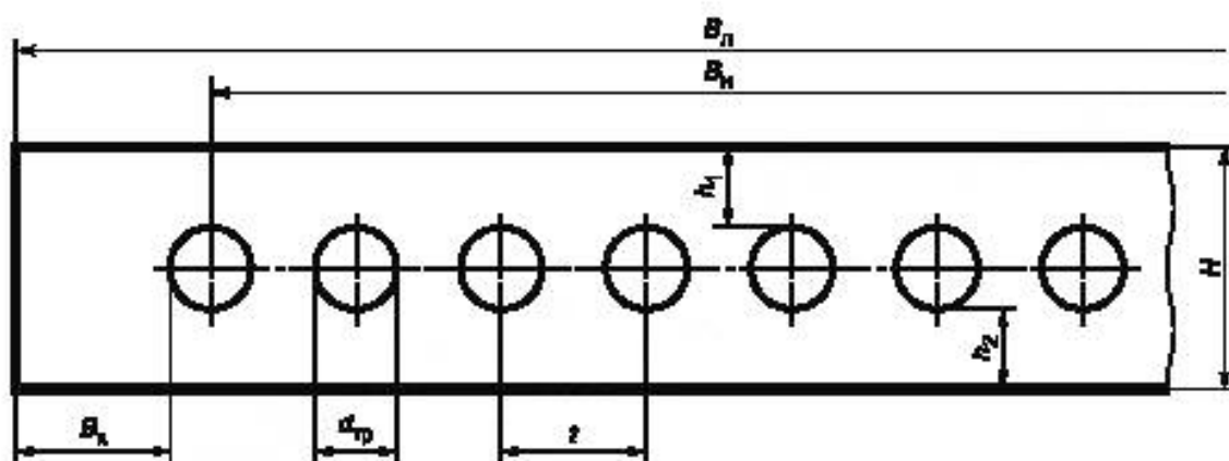
а — Бестканевая конструкция (РТЛ)
