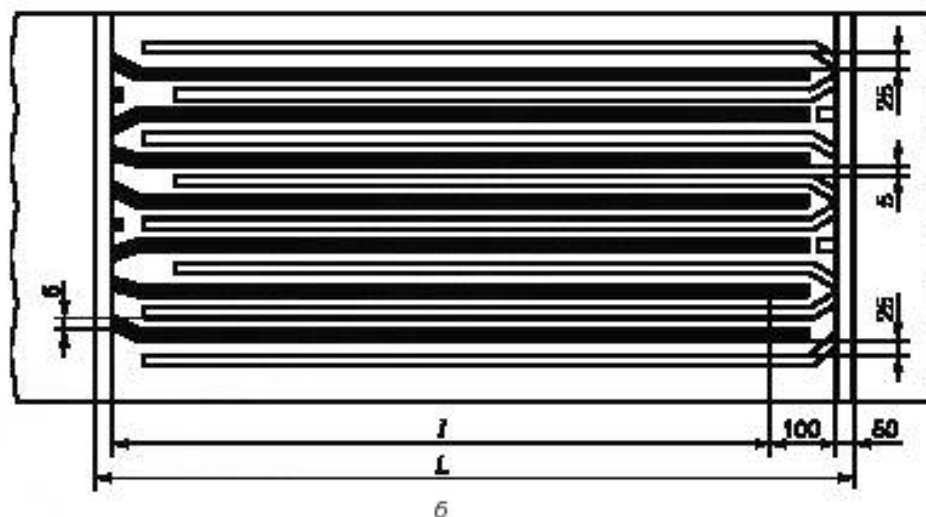
Рисунок Б.1. лист 2
