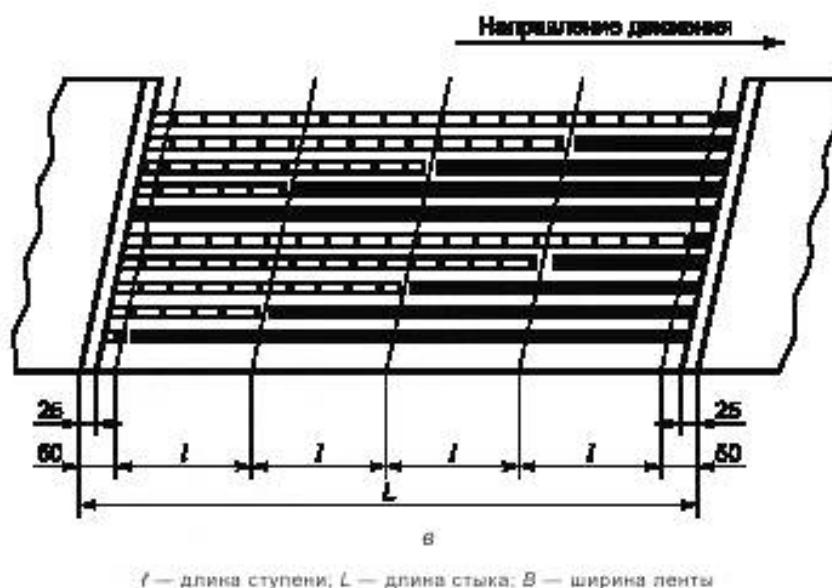
Рисунок Б.2, лист 2
