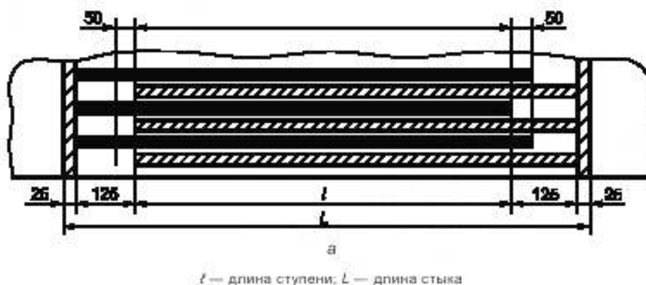
Рисунок Б.1 — Одноступенчатые схемы стыковки
