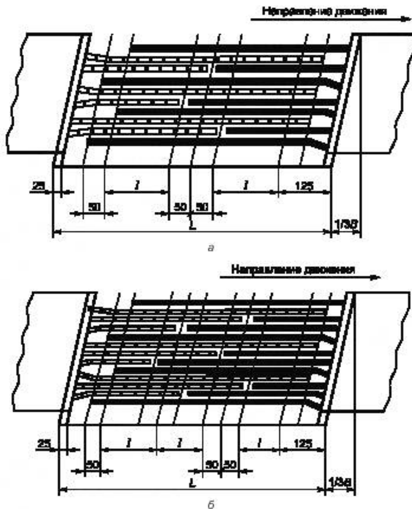
Рисунок Б.1. лист 2
