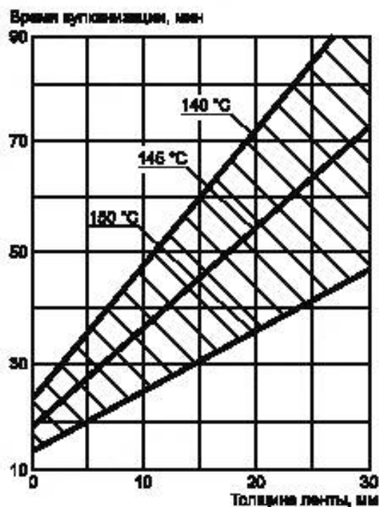
Рисунок Б.3 — Режим вулканизации стыка ленты
