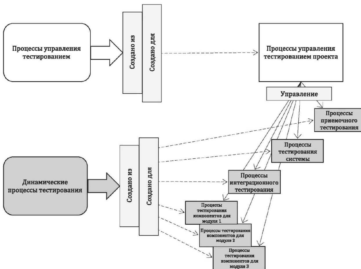
Рисунок 5 — Создание нескольких экземпляров наборов процессов динамического тестирования
