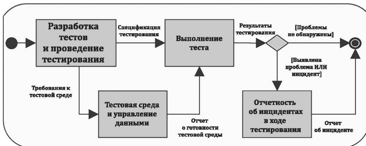
Рисунок 4 — Процессы динамического тестирования
