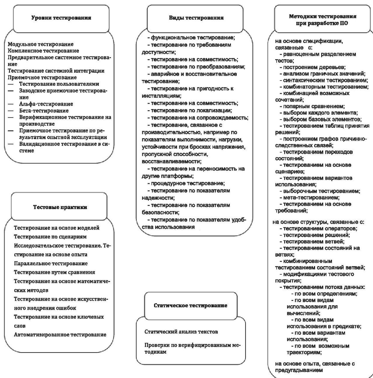
Рисунок 1 — Примеры возможных типовых подходов к тестированию ПО
