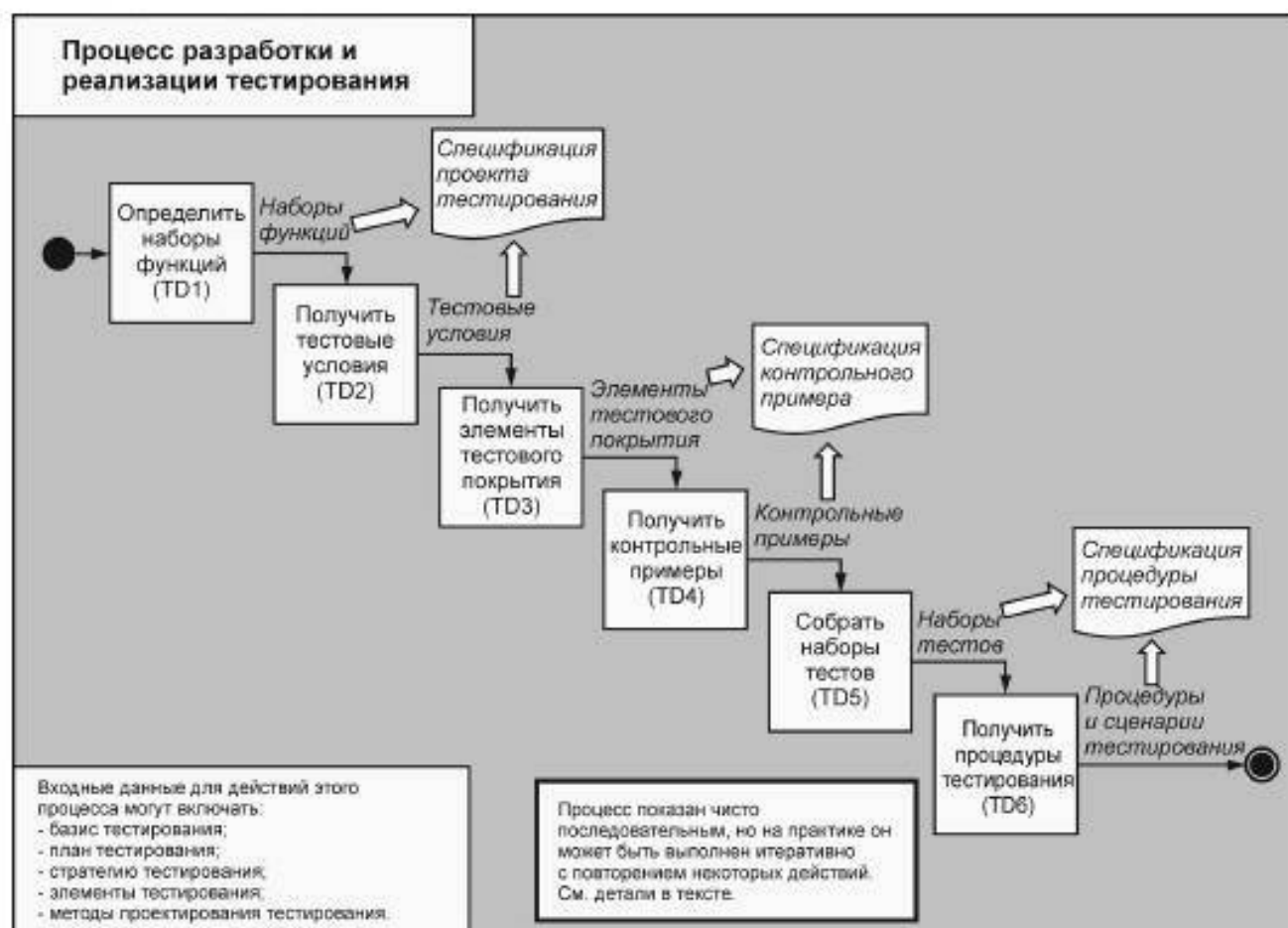
Рисунок 10 — Процесс Разработки и Реализации Тестирования
