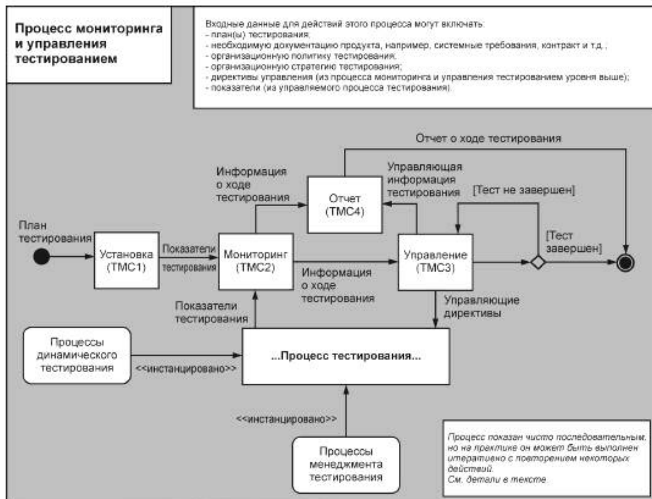
Рисунок 7 — Процесс Мониторинга и Управления Тестированием
