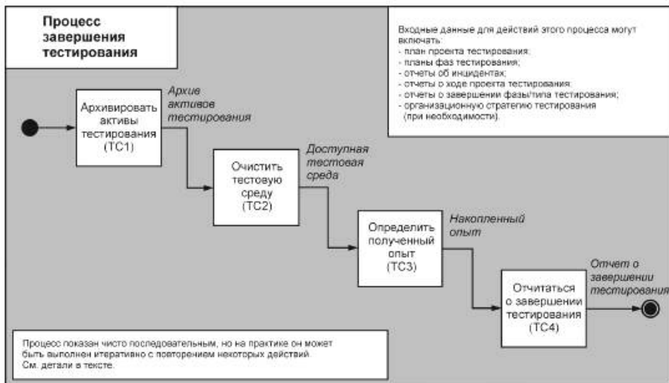
Рисунок 8 — Процесс Завершения Тестирования
