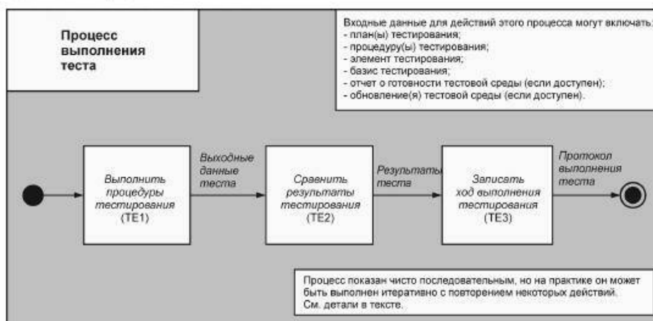
Рисунок 12 — Процесс Выполнения Теста
