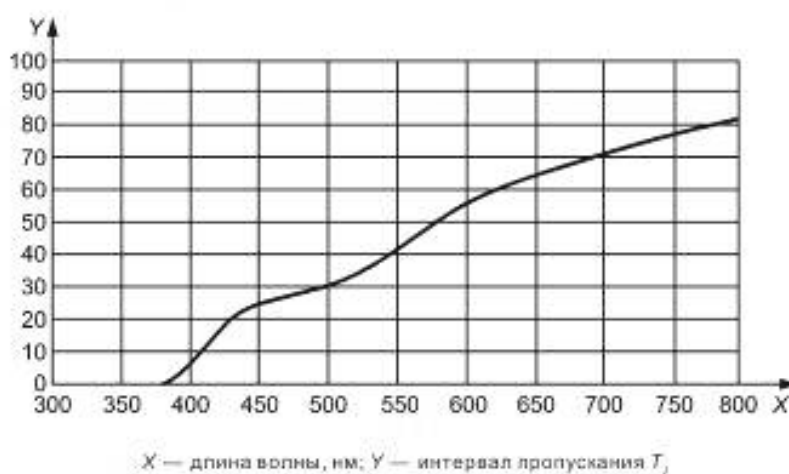
Рисунок 6 — Внутреннее пропускание цветопреобразующего фильтра
