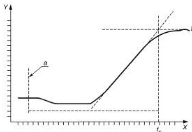
Рисунок 5 — Метод определения времени отверждения
