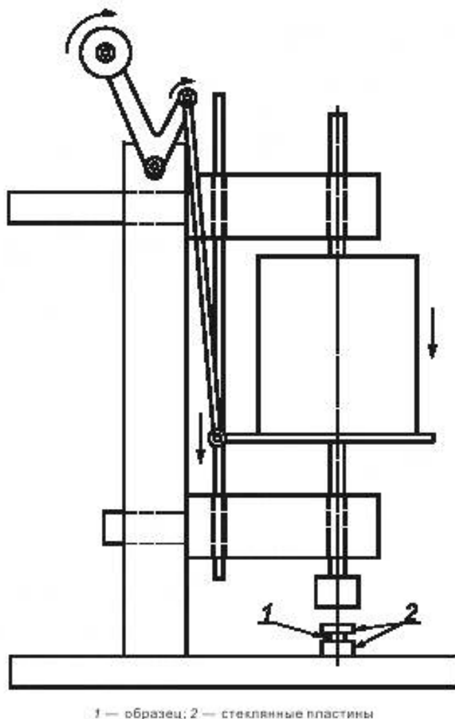
Рисунок 1 — Нагружающее устройство
