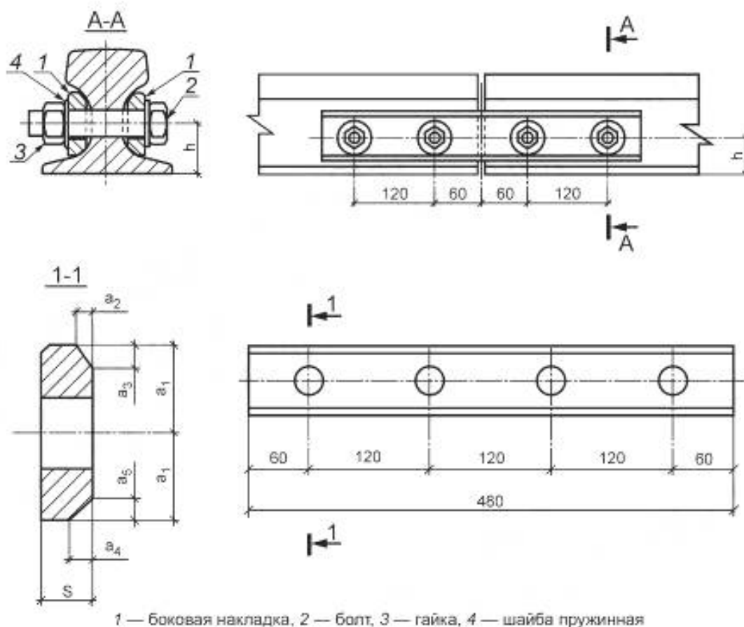
Рисунок А.2 — Четырехдырные накладки для крановых рельсов типа КР (размеры в мм)
