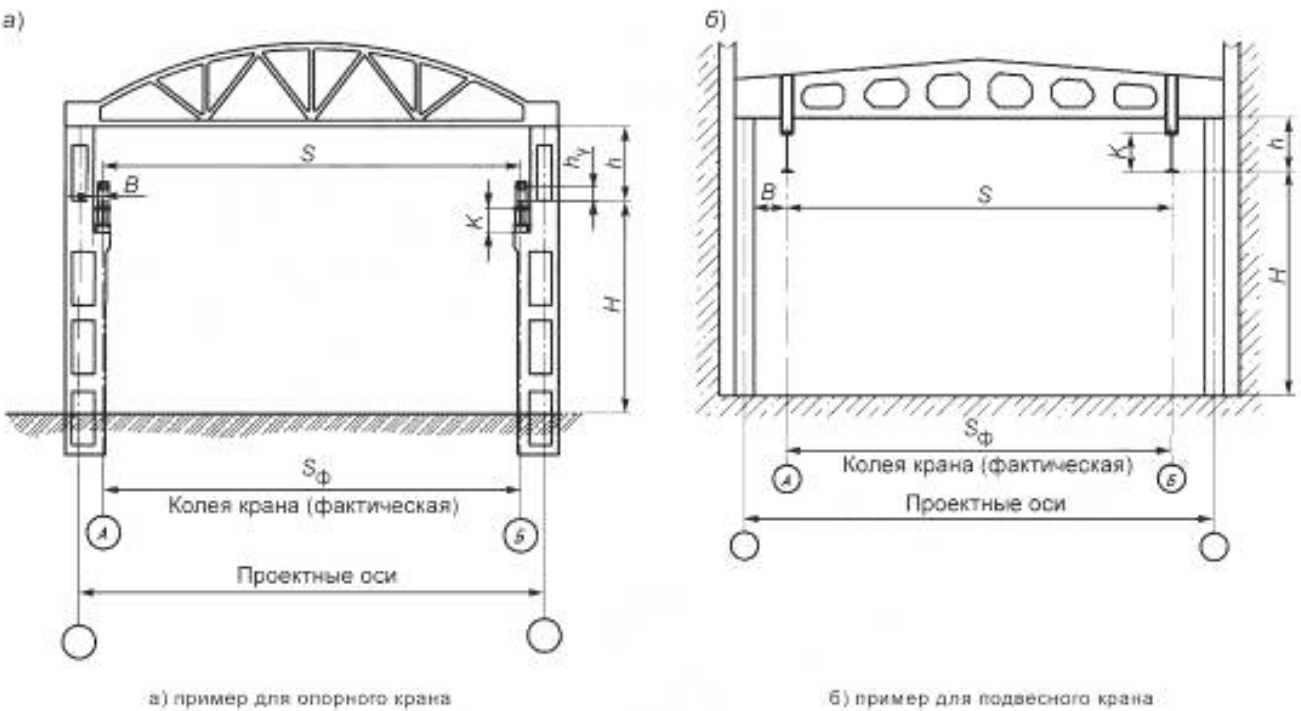
Рисунок 1 — Поперечный разрез пролета
