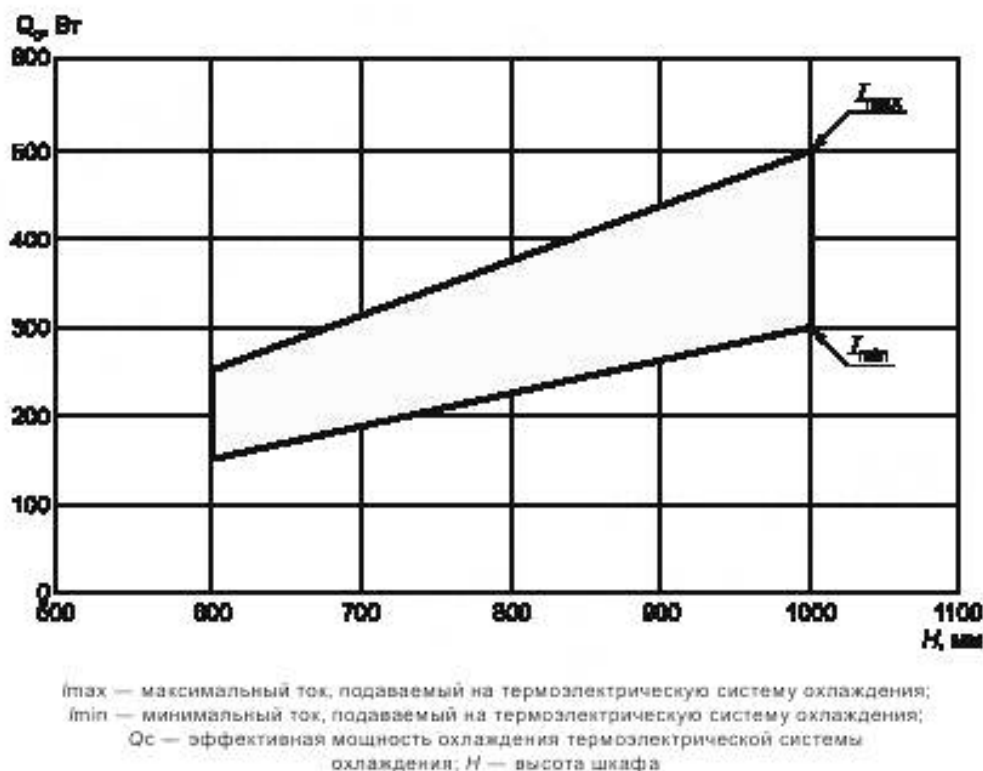
Рисунок 7 — Оценка эффективности термоэлектрической системы охлаждения, установленной сверху
