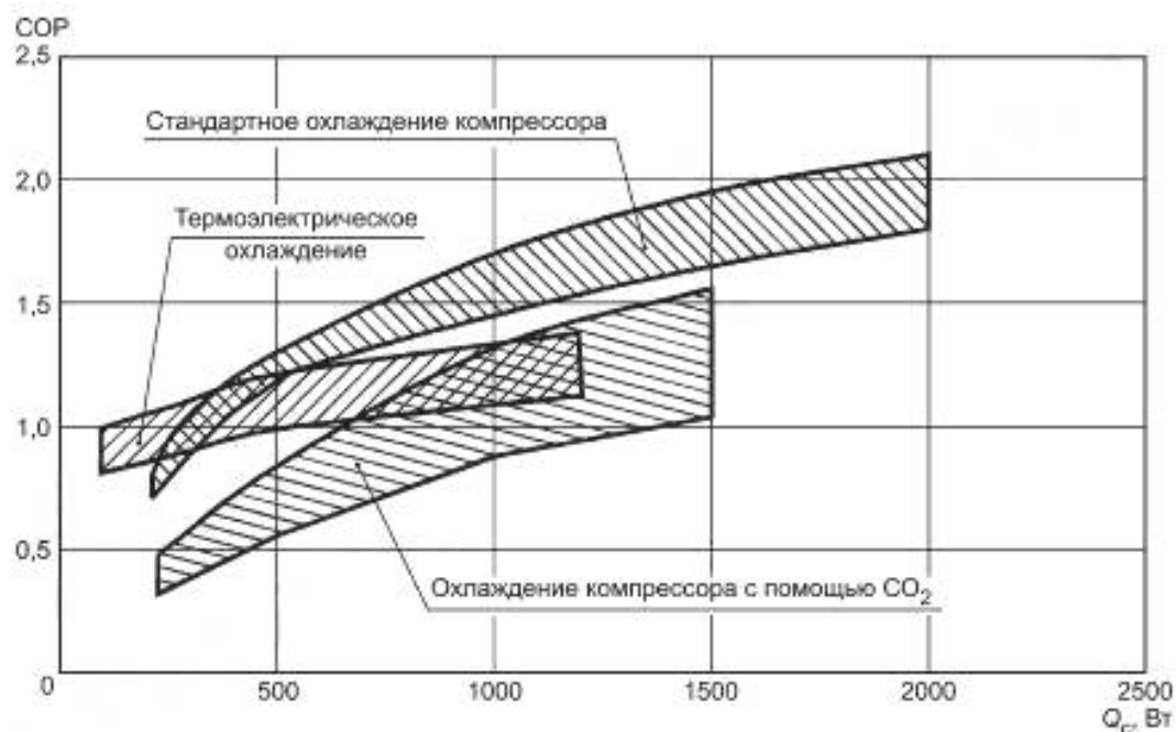
Рисунок А.4 — Коэффициент эффективности, зависящий от мощности охлаждения в пограничных условиях T_d = 50^\circ\text{C}
