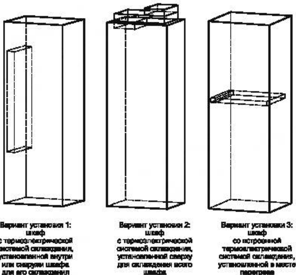
Рисунок 1 — Общее представление расположения системы охлаждения
