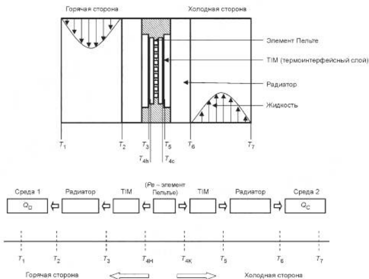
Рисунок А.6 — Тепловое сопротивление термоэлектрической системы охлаждения
