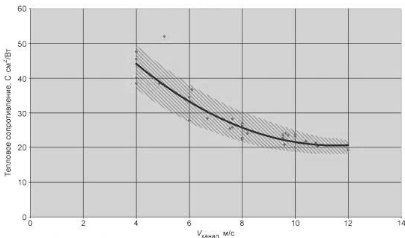
Рисунок А.8 — Пример теплового сопротивления между воздухом и радиатором как функция скорости воздушного потока
