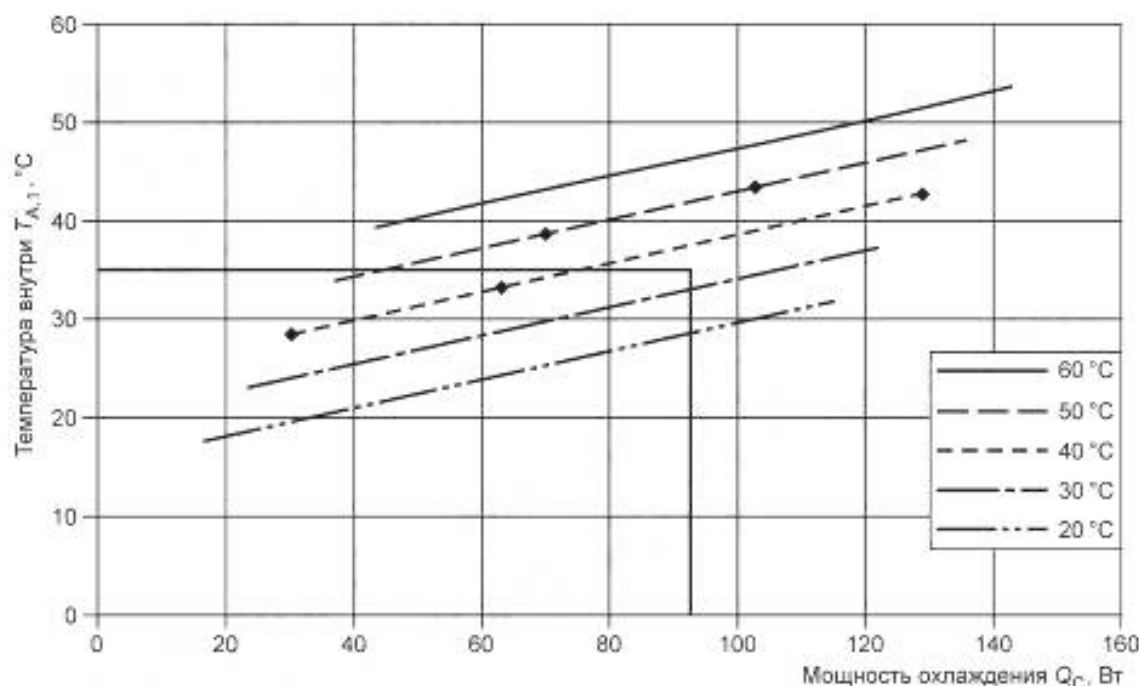
Рисунок 5 — Результаты измерений
