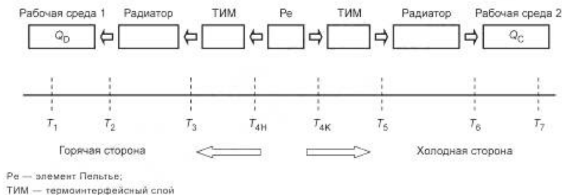
Рисунок 2 — Тепловые сопротивления
