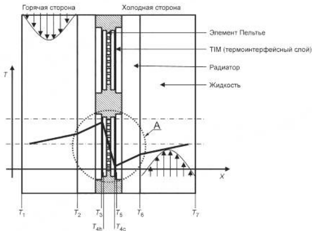
Рисунок 1, лист 1 — Принцип действия термоэлектрической системы охлаждения
