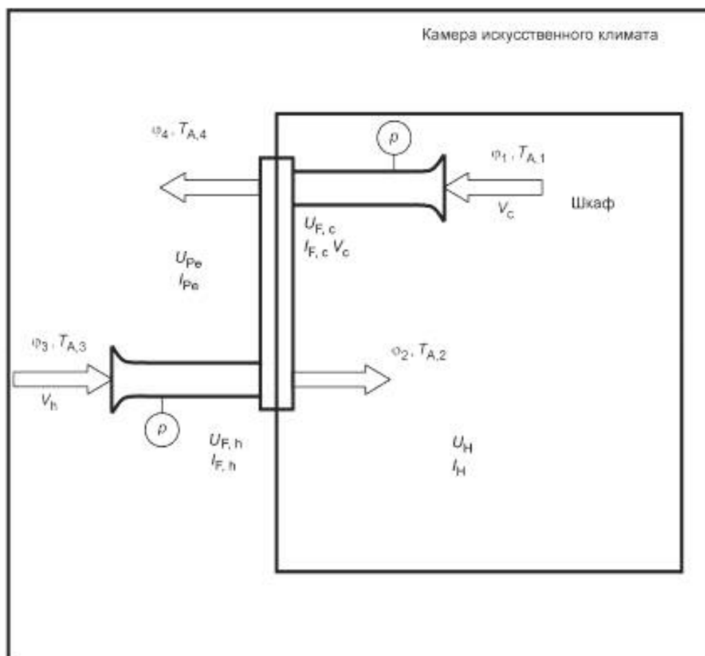
Рисунок 4 – Схема измерительной установки
