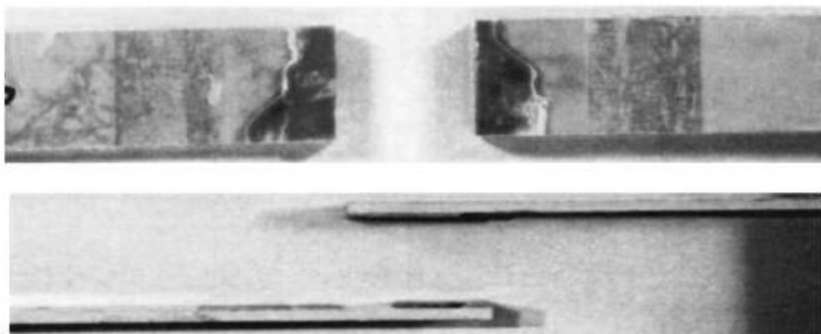
Рисунок А.10 — Адгезионное разрушение
