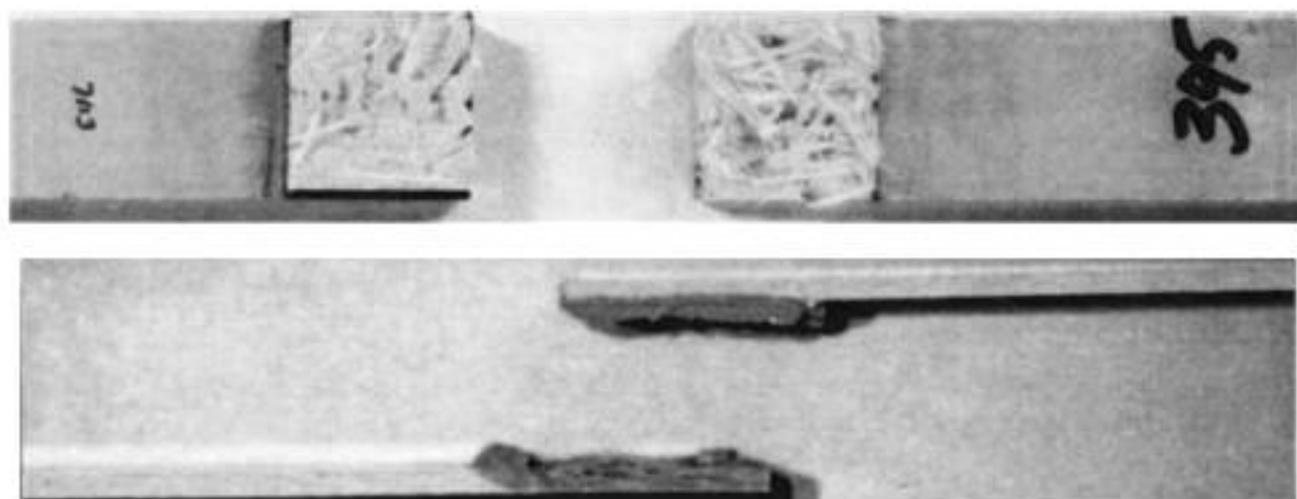
Рисунок А.13 — Разрушение из-за разрыва волокон
