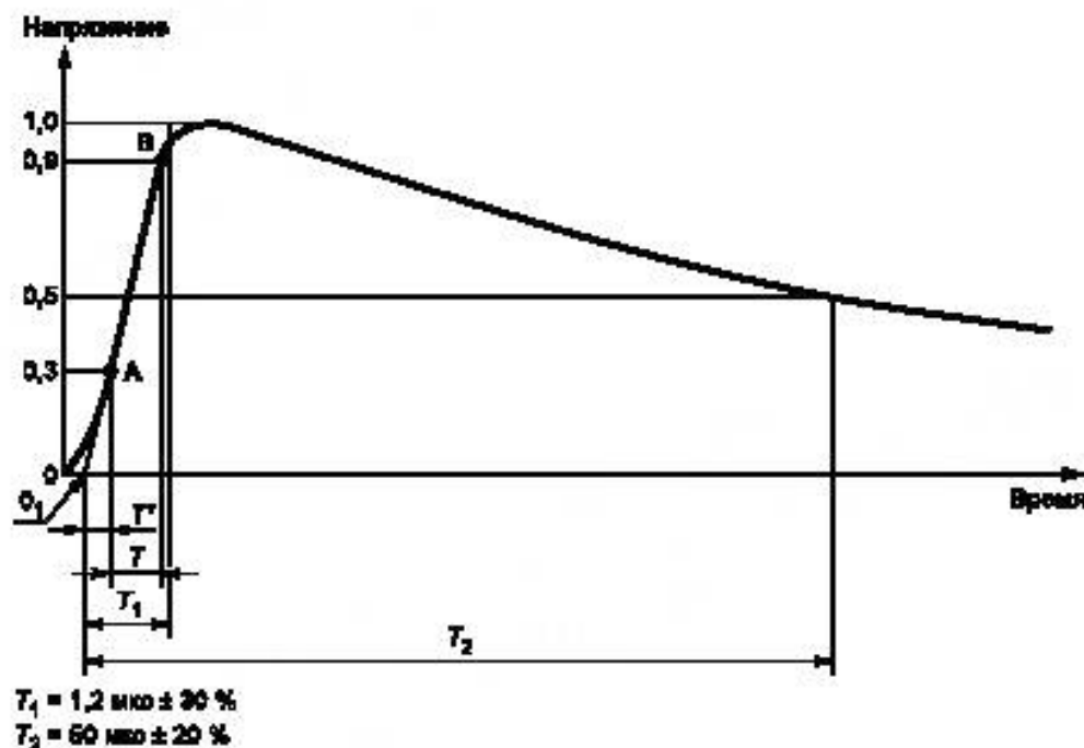
Рисунок 7 — Форма импульса испытательного напряжения 1,2/50
