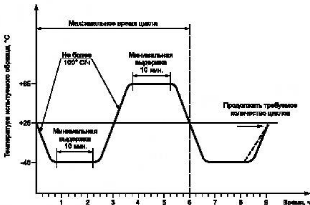
Рисунок 4 — Профиль изменения температуры при термоциклировании
