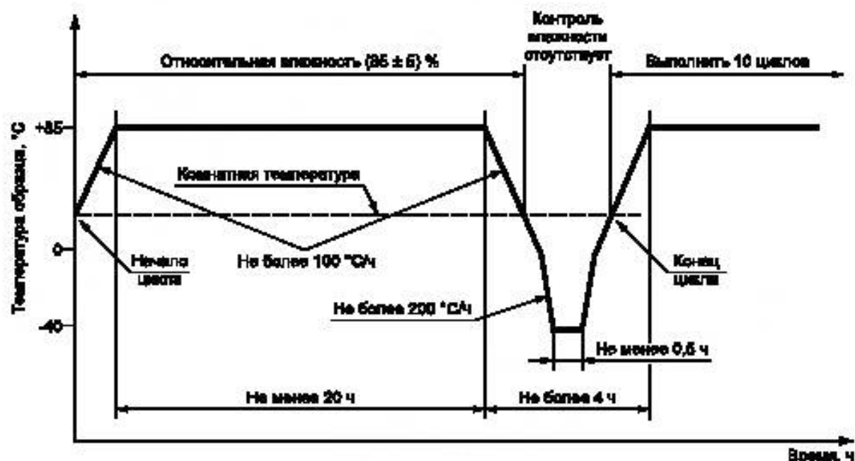
Рисунок 5 — Цикл термоциклирования при высокой влажности
