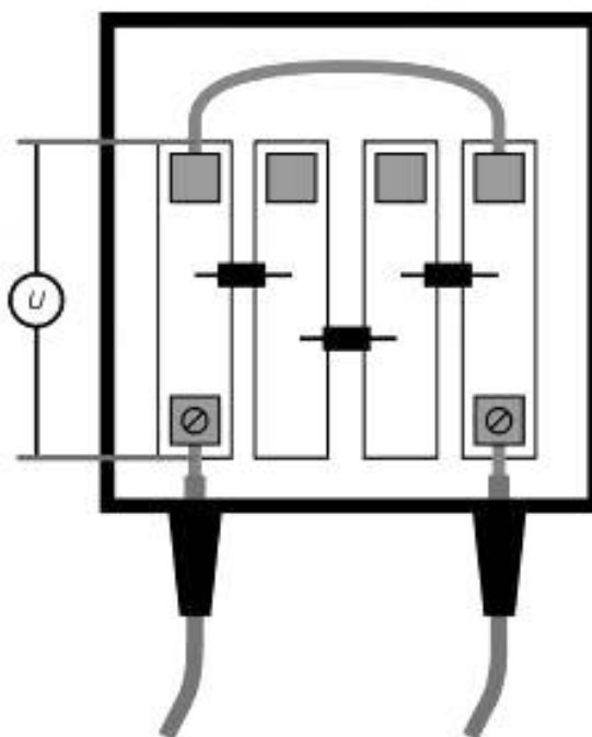
Рисунок 6 — Пример измерения напряжения для определения сопротивления контактов
