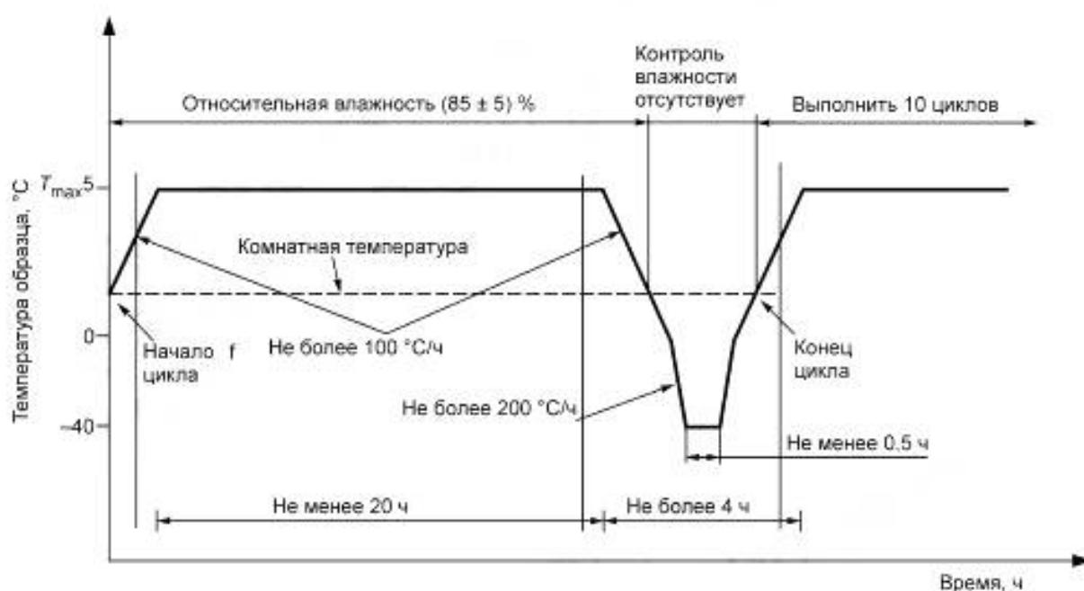
Рисунок 4 — Цикл термоциклирования при высокой влажности
